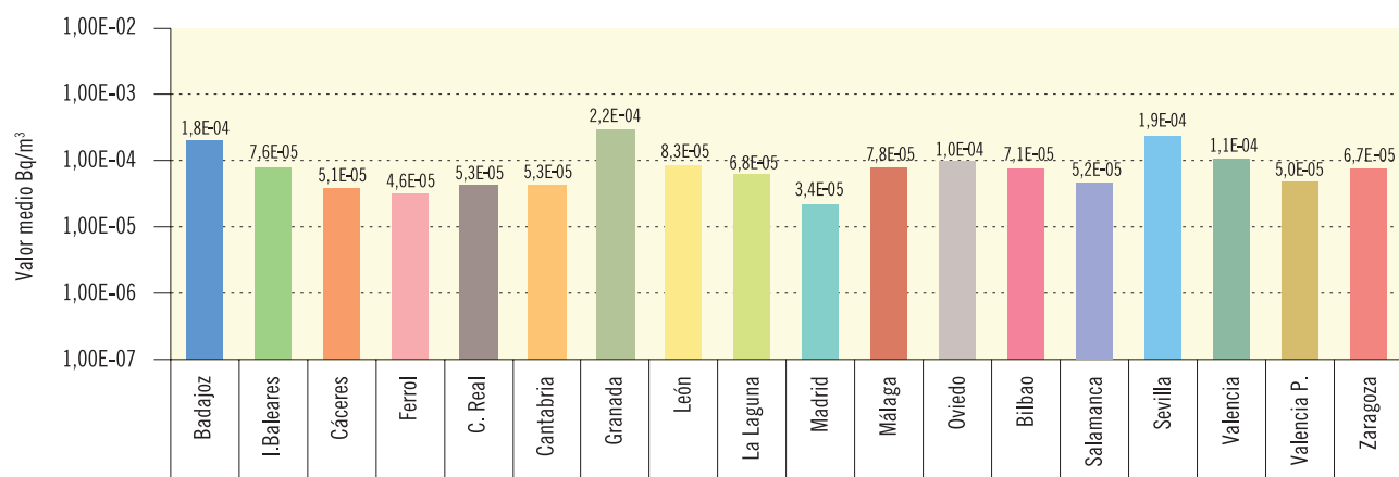
Figura 3.2b. Partículas de polvo en aire. Concentración del índice de actividad alfa total (Bq/m³)
