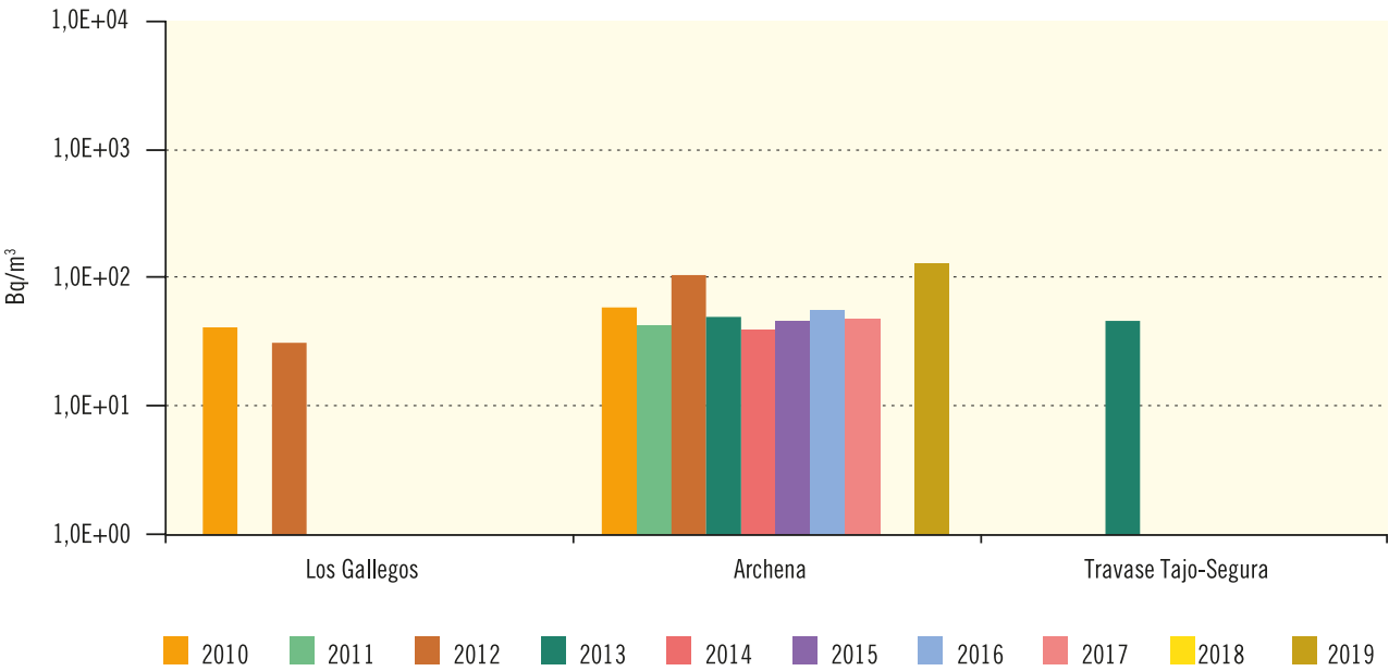
Figura 3.48. Río Segura Evolución temporal del índice de actividad beta resto
