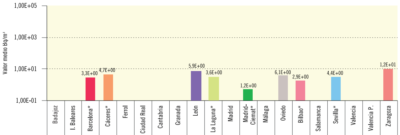
Figura 3.13b. Agua potable. Concentración de actividad de Sr-90 (Bq/m³)
