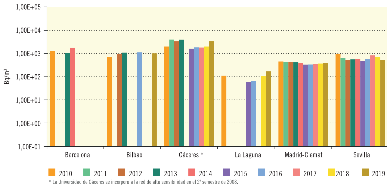
Figura 3.14a. Red de alta sensibilidad. Agua potable
