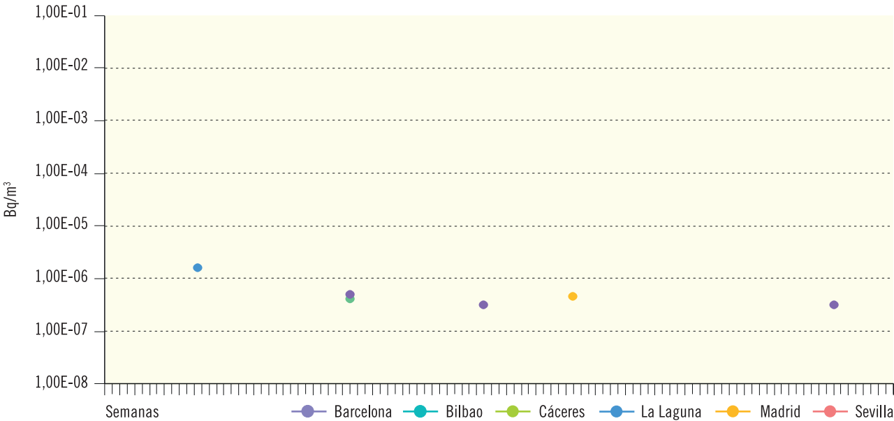
Figura 3.5b. Red de alta sensibilidad. Partículas de Polvo en aire. Muestreador alto flujo Concentración de actividad de Cs-137 (Bq/m³). Valores de la campaña de 2019
