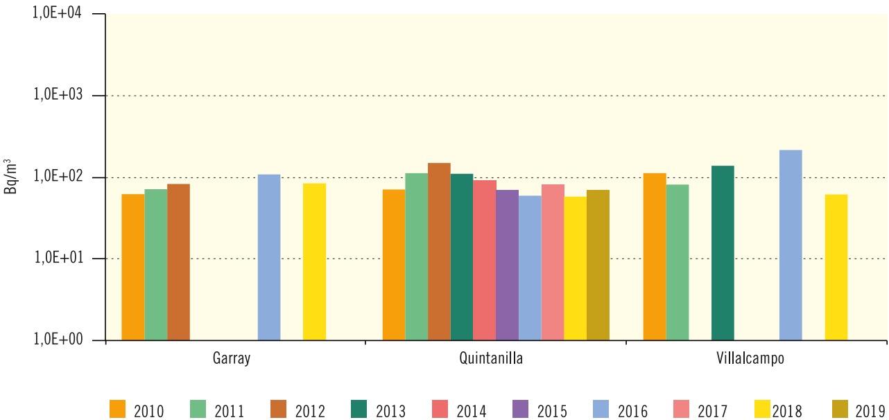
Figura 3.32. Río Duero Evolución temporal del índice de actividad beta resto
