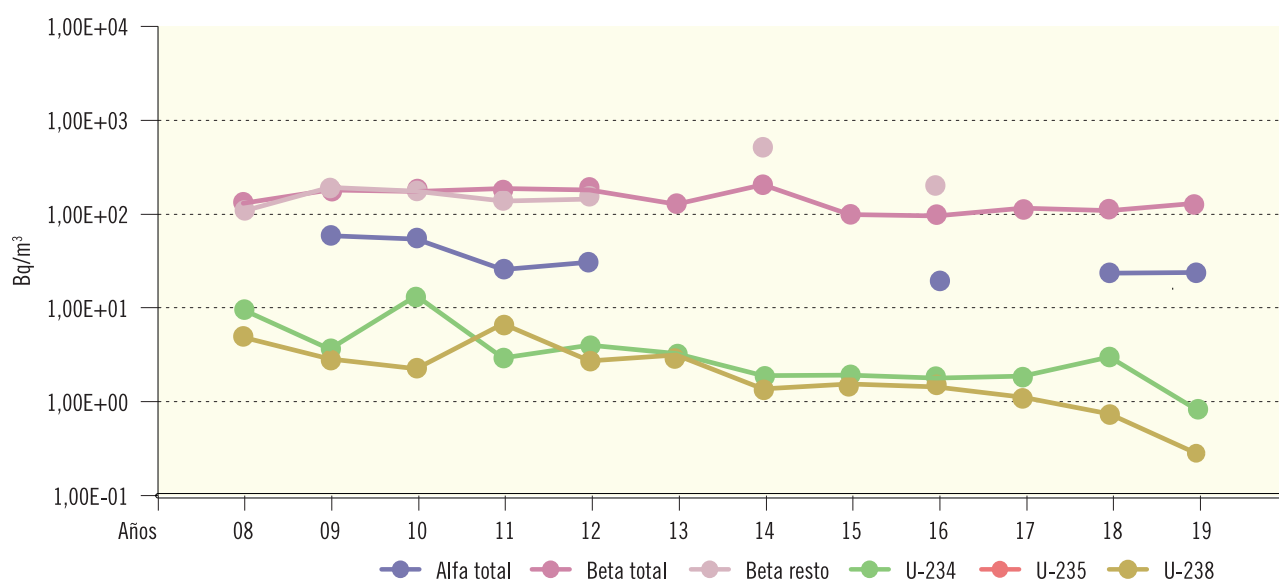
Figura 2.40. Juzbado. Agua potable. Valores de concentración de actividad (Bq/m³) Evolución temporal valores medios
