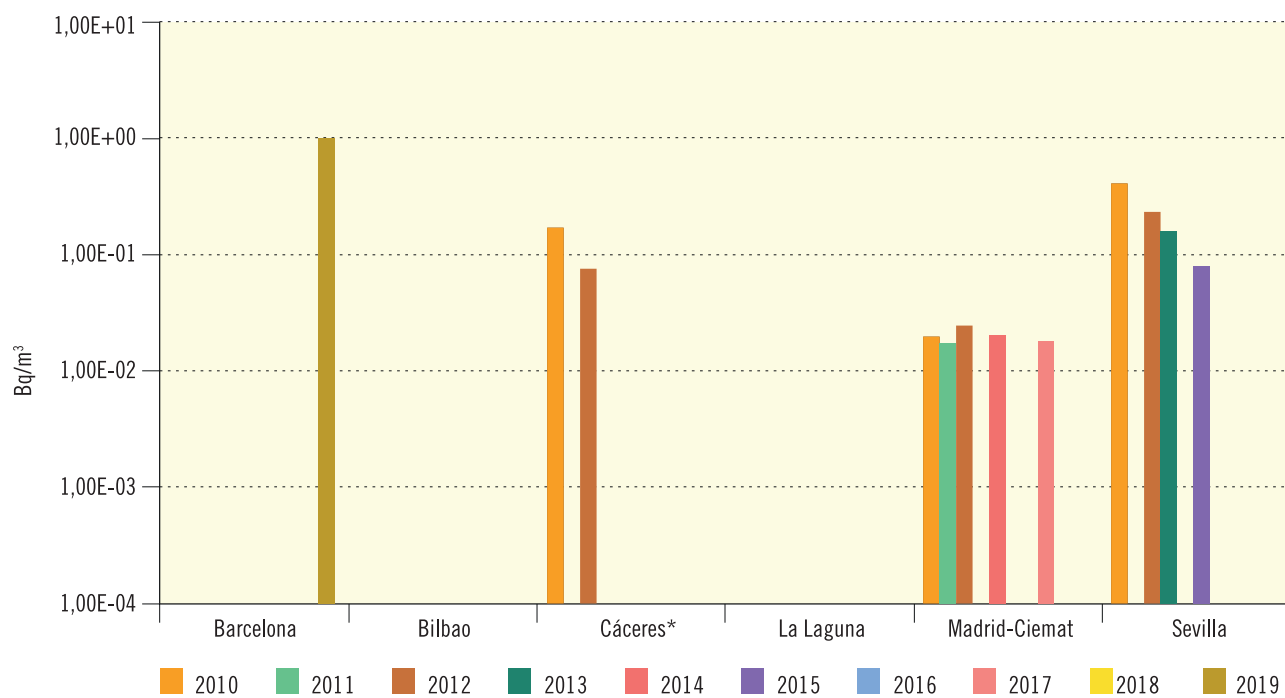
Figura 3.15a. Red de alta sensibilidad. Agua potable
