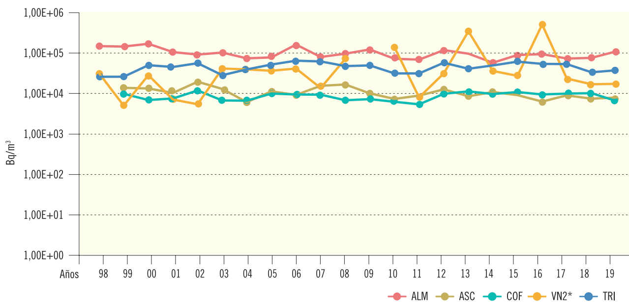
Figura 2.14a. Agua superficial. Evolución temporal de la concentración de actividad de H-3
