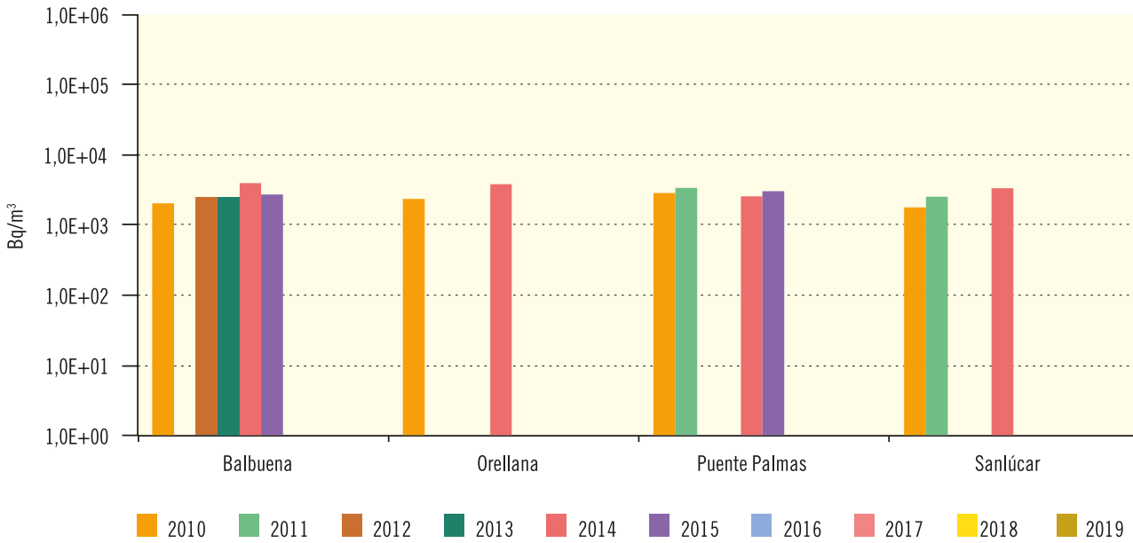
Figura 3.41. Río Guadiana Evolución temporal de concentración de actividad de H-3
