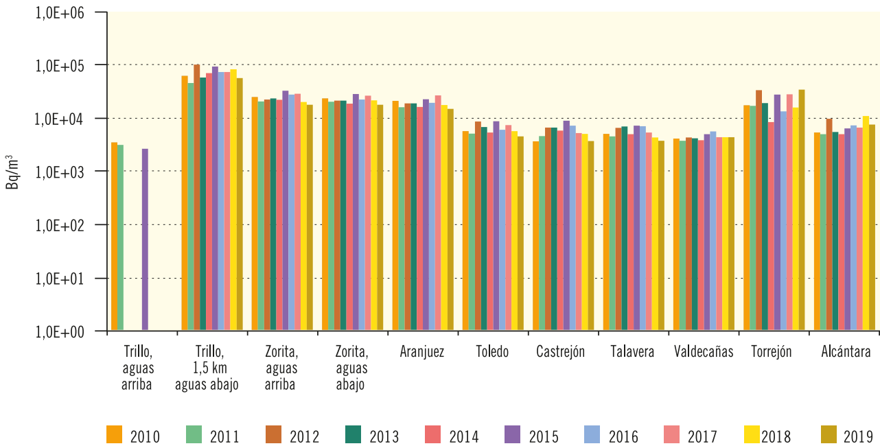
Figura 3.37. Río Tajo Evolución temporal de concentración de actividad de H-3
