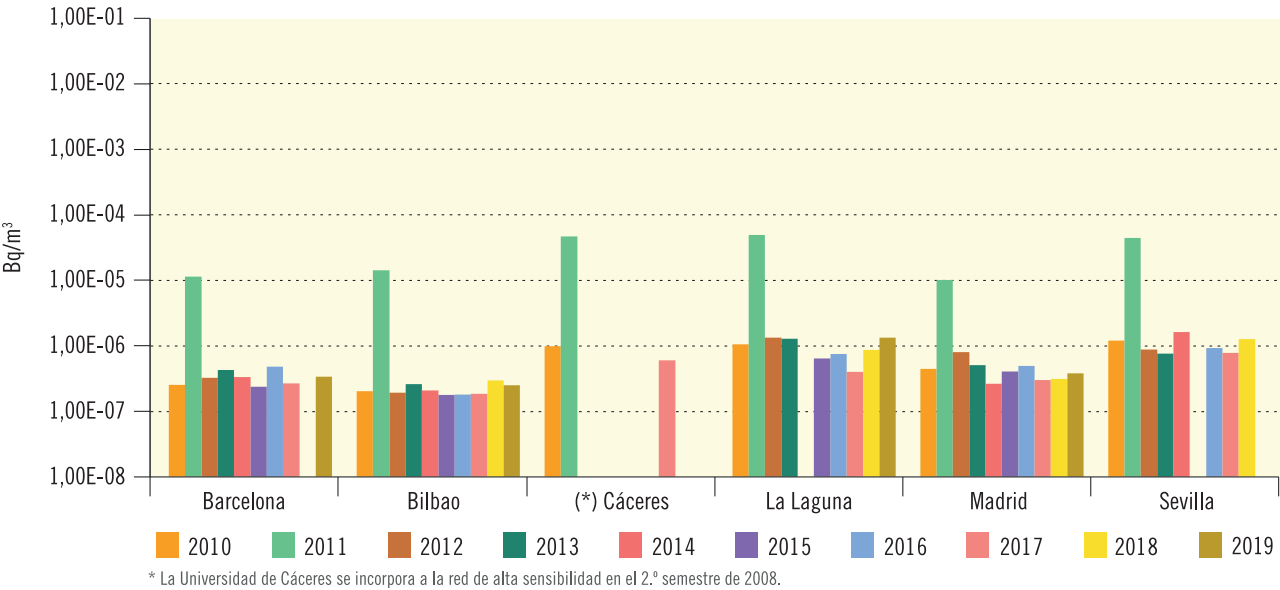
Figura 3.5a. Red de alta sensibilidad. Partículas de polvo en aire. Muestreador alto flujo Evolución temporal de la concentración de actividad de Cs-137
