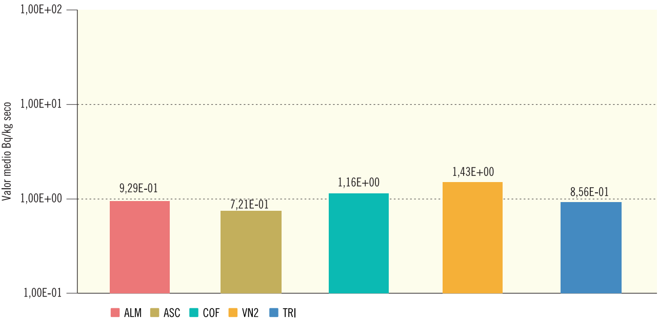
Figura 2.10b. Suelo. Concentración de actividad de Sr-90 (Bq/kg seco) Valores de la campaña de 2019
