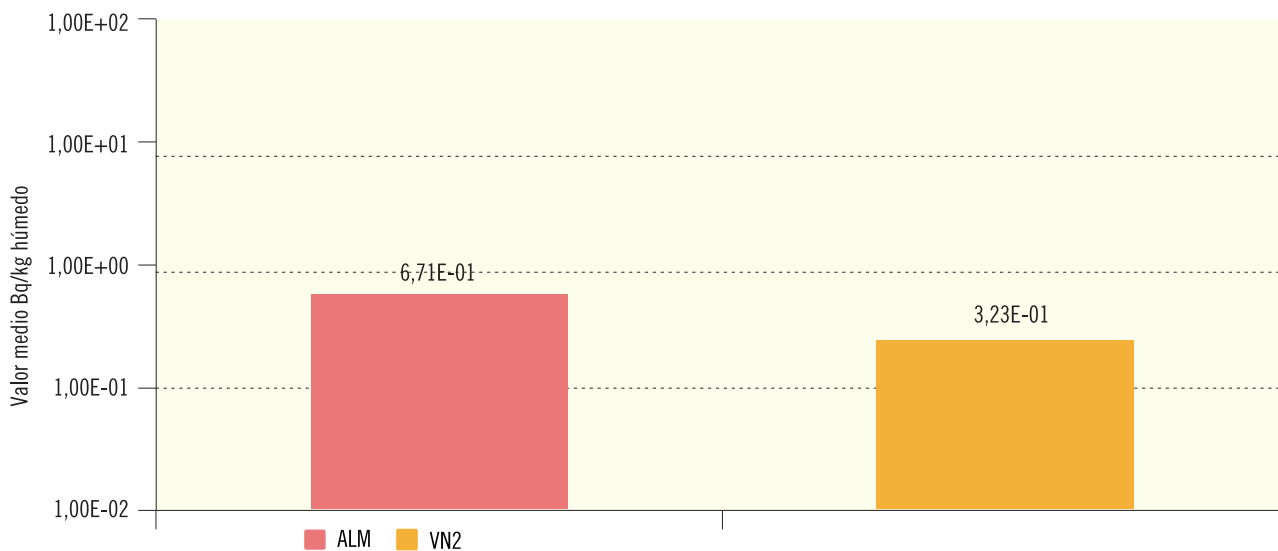
Figura 2.29b. Consumo animal. Concentración de actividad de Sr-90 (Bq/kg húmedo)
