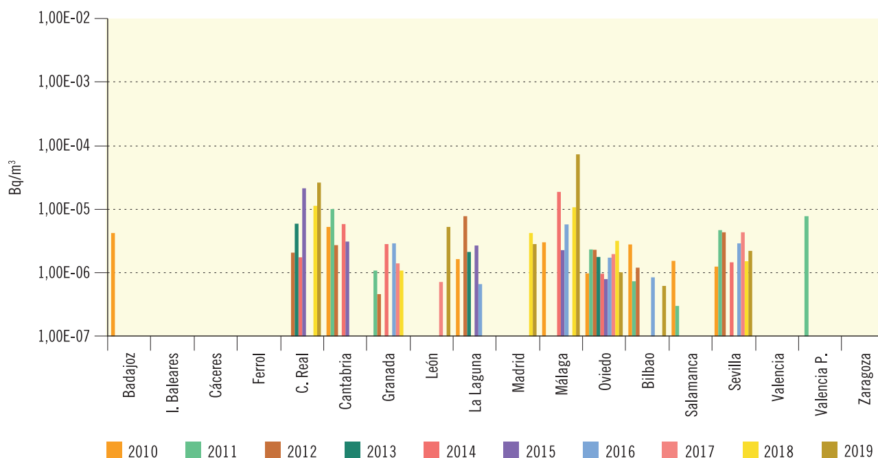
Figura 3.4a. Partículas de polvo en aire
