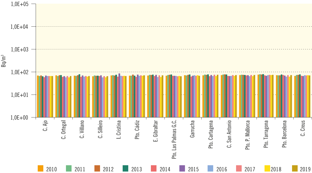
Figura 3.64a. Agua de mar Evolución temporal del índice de actividad alfa total
