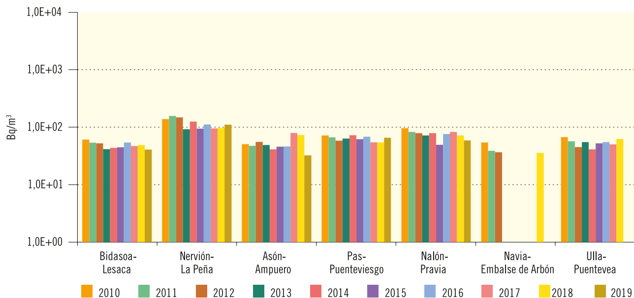
Figura 3.23. Cuencas del norte de España
