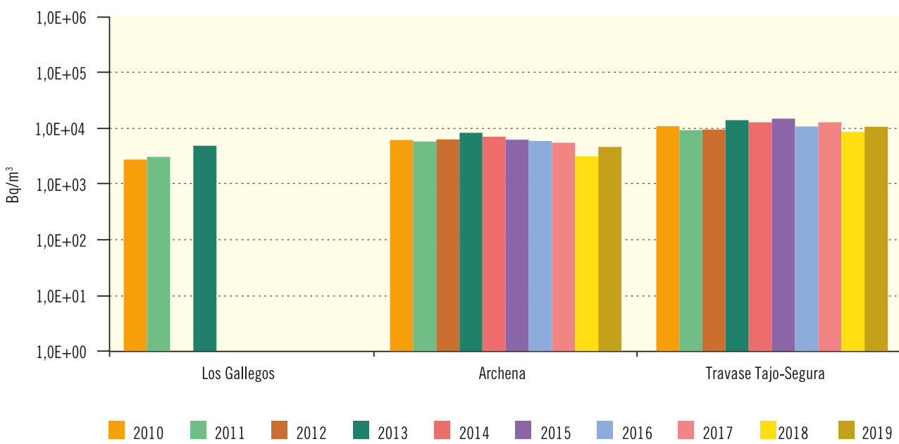
Figura 3.49. Río Segura Evolución temporal de la concentración de actividad de H-3
