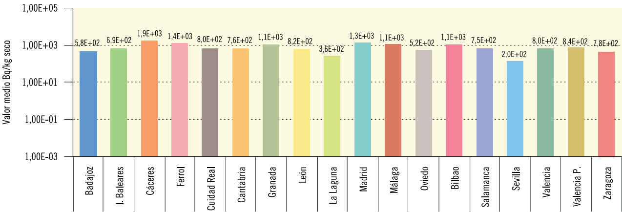
Figura 3.7b. Suelo. Concentración del índice de actividad beta total (Bq/kg seco) Valores de la campaña de 2019
