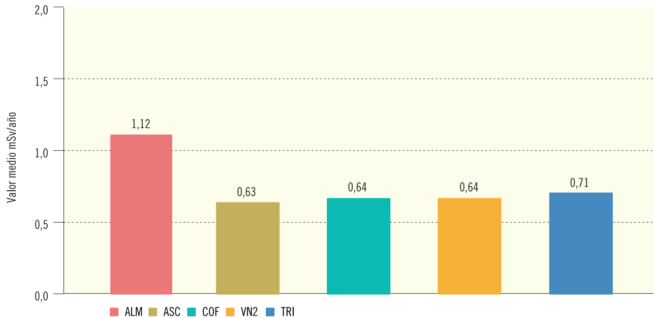
Figura 2.9b. Radiación directa. Dosis integrada (DTL). (mSv/año) Valores de la campaña de 2019
