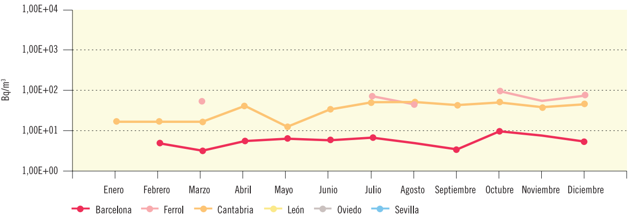
Figura 3.17b. Leche, Concentración de actividad de Cs-137 (Bq/m3) Valores de la campaña 2019
