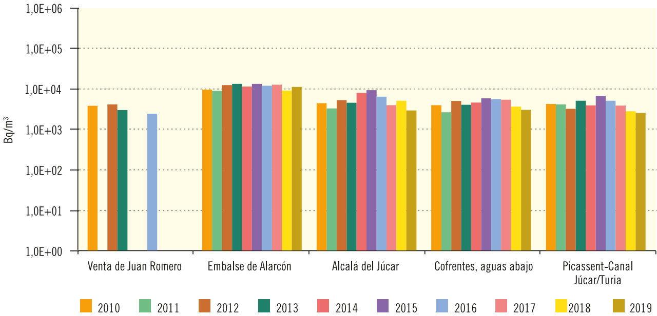
Figura 3.53. Río Júcar Evolución temporal de la concentración de actividad de H-3
