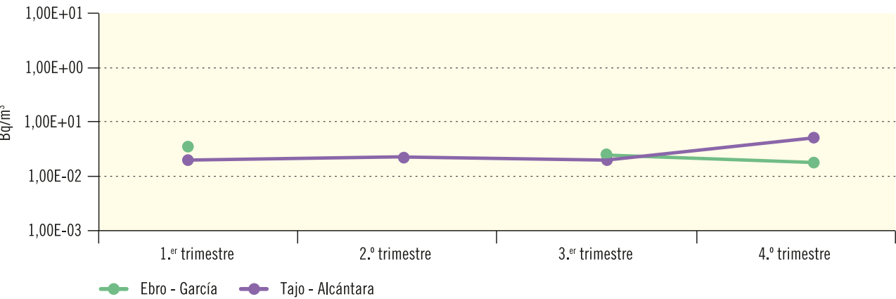
Figura 3.62b. Red de alta sensibilidad. Agua superficial. Concentración de actividad de Cs-137 (Bq/m³) Valores de la campaña 2019
