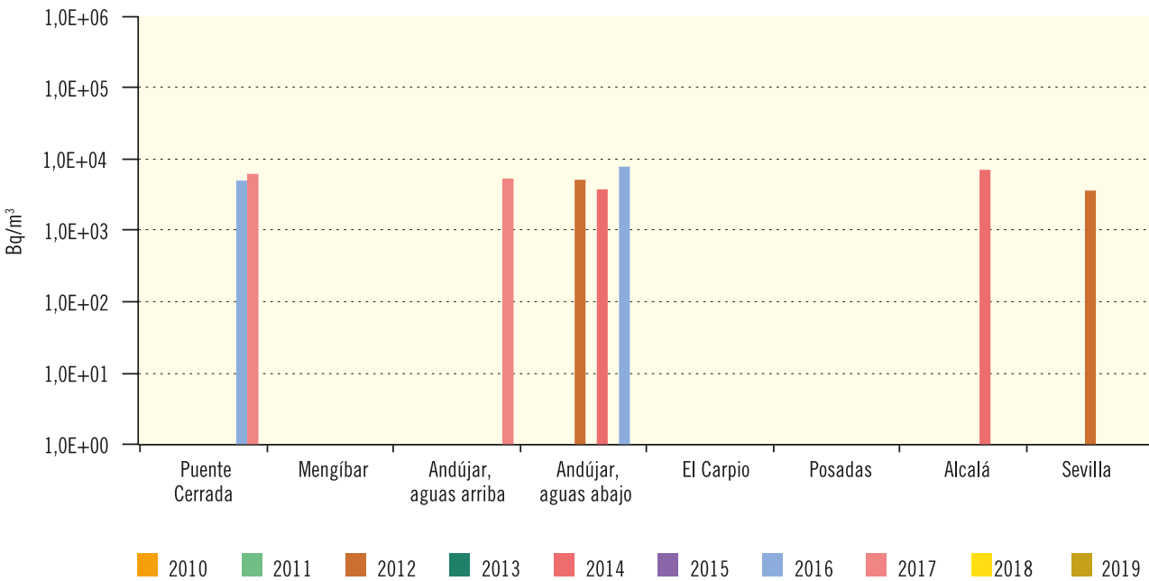
Figura 3.45. Río Guadalquivir Evolución temporal de la concentración de actividad de H-3
