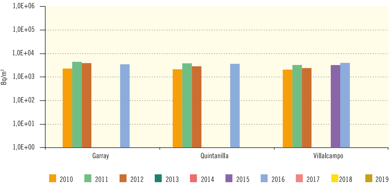
Figura 3.33. Río Duero Evolución temporal de concentración de actividad de H-3
