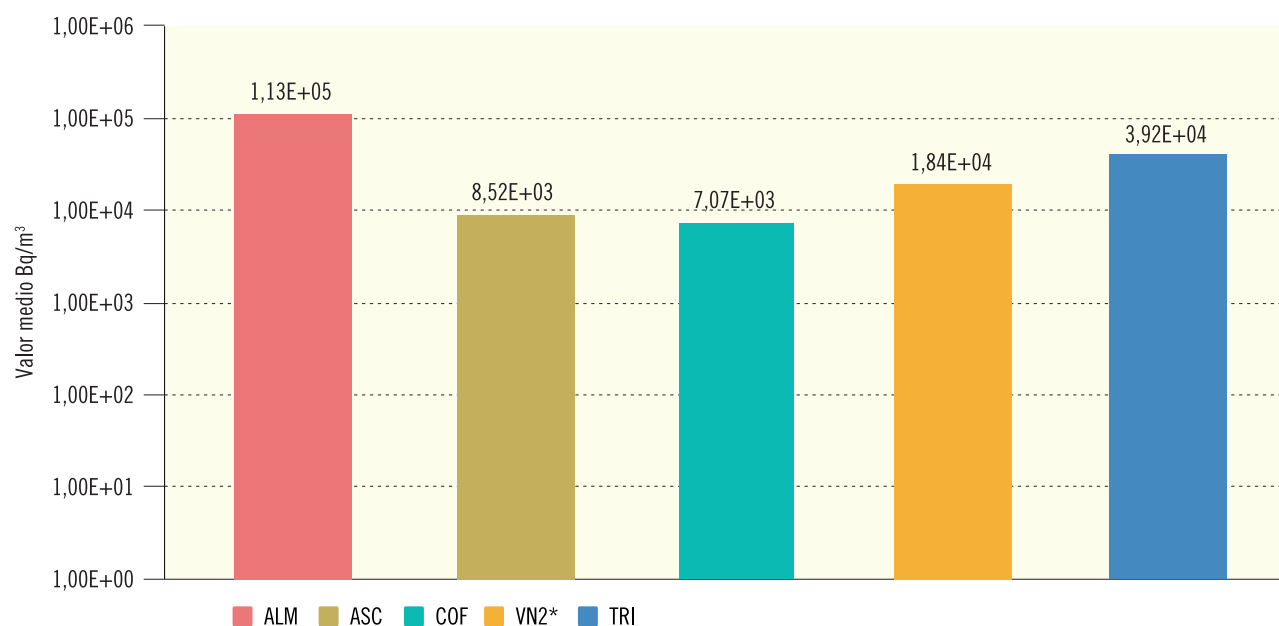
Figura 2.14b. Agua superficial. Concentración de actividad de H-3 (Bq/m³)
