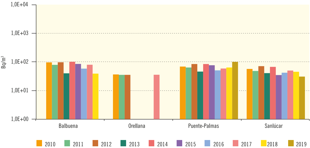
Figura 3.40. Río Guadiana Evolución temporal del índice de actividad beta resto
