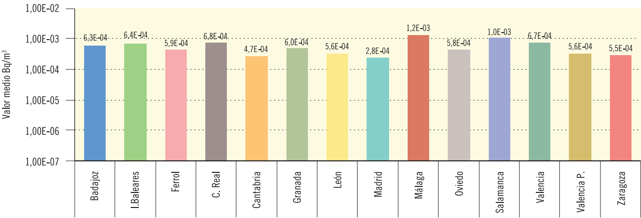
Figura 3.3b. Partículas de polvo en aire. Concentración del índice de actividad beta total (Bq/m³) Valores de la campaña de 2019
