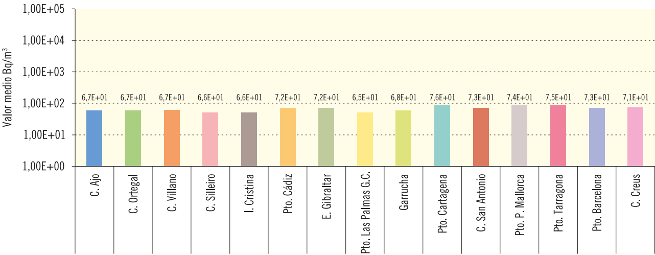
Figura 3.64b. Agua de mar. Concentración del índice de actividad alfa total (Bq/m³) Valores de la campaña de 2019
