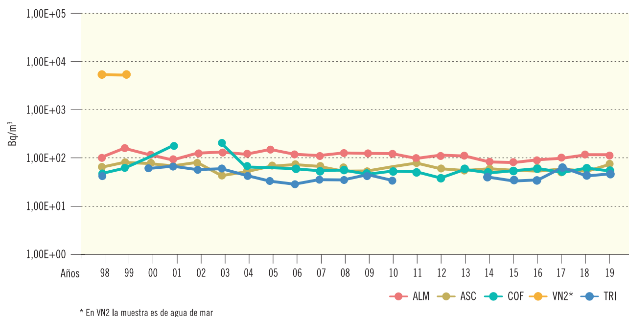
Figura 2.13a. Agua superficial. Evolución temporal del índice de actividad beta resto
