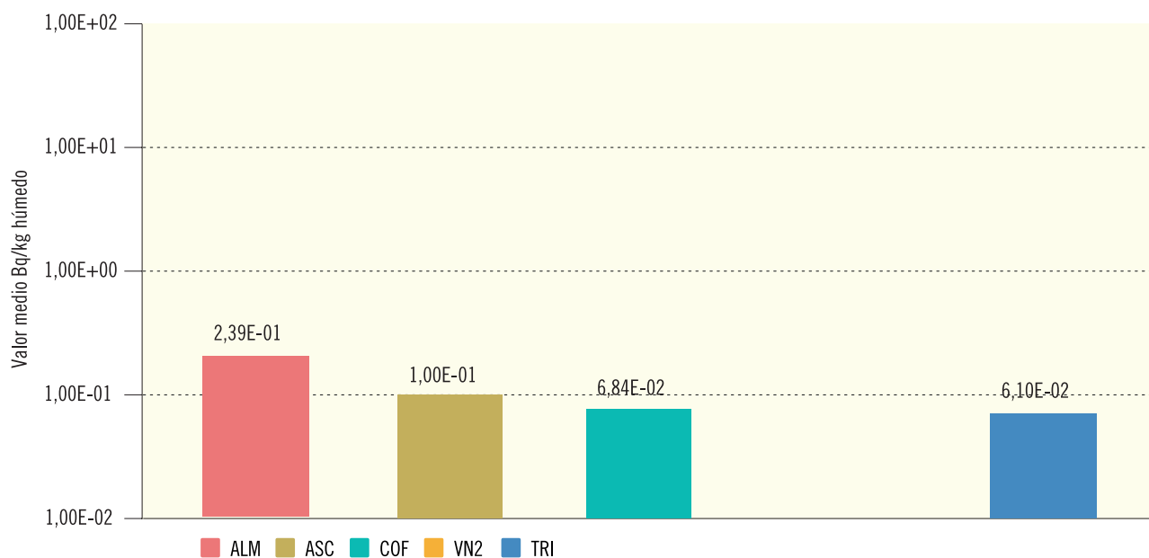
Figura 2.27b. Vegetales de hoja ancha. Concentración de actividad de Sr-90 (Bq/kg húmedo)
