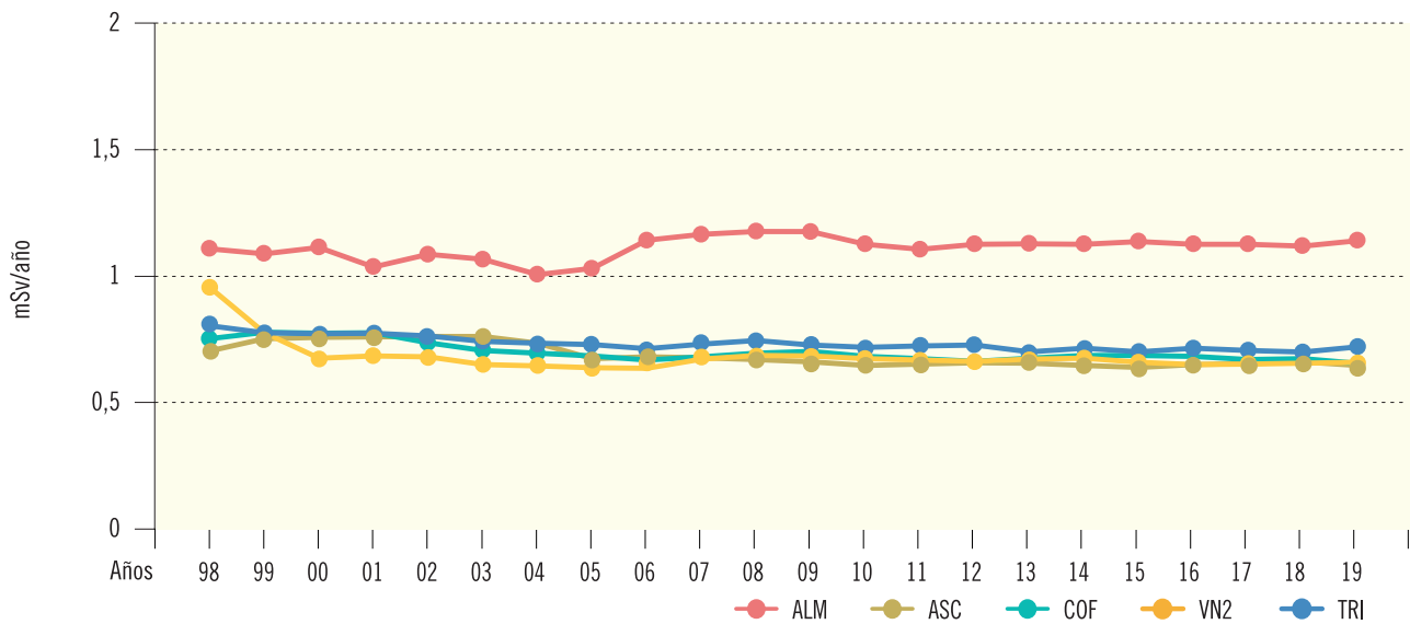
Figura 2.9a. Radiación directa. Dosis integrada (DTL) Valores medios en la zona vigilada
