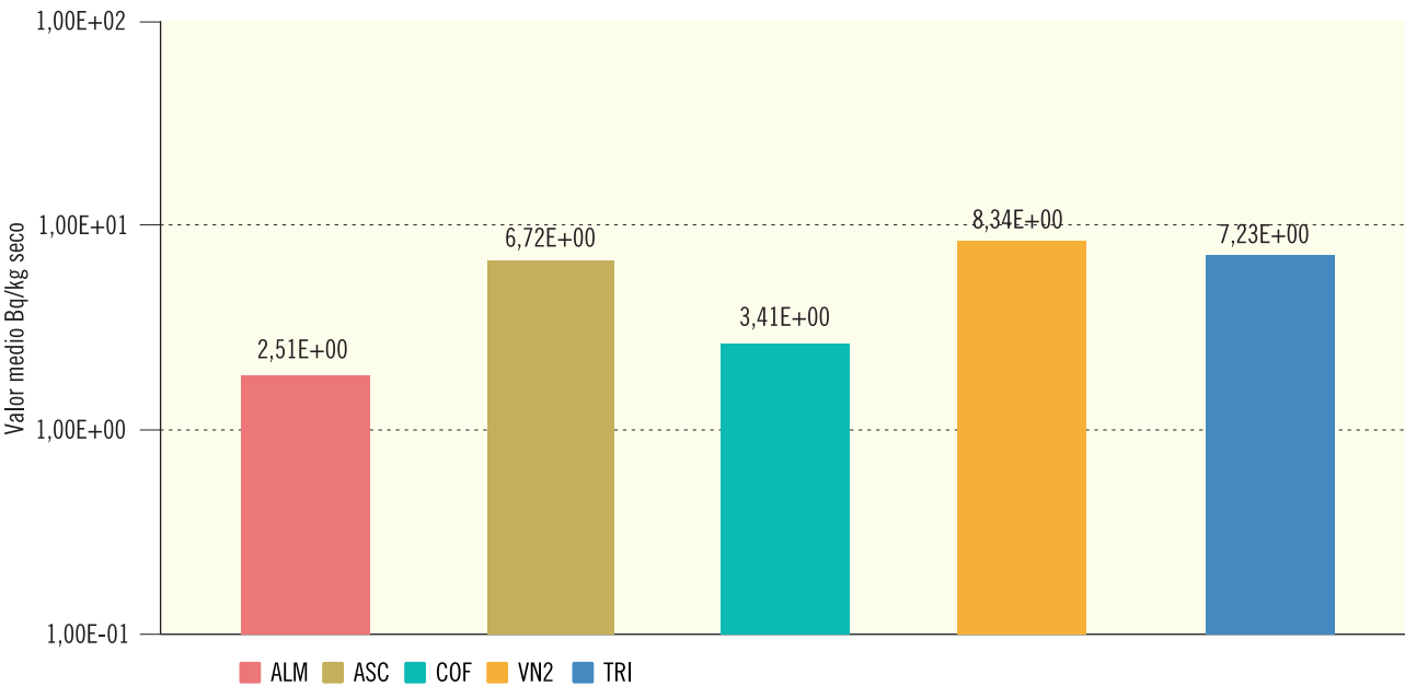
Figura 2.11b. Suelo. Concentración de actividad de Cs-137 Valores de la campaña de 2019
