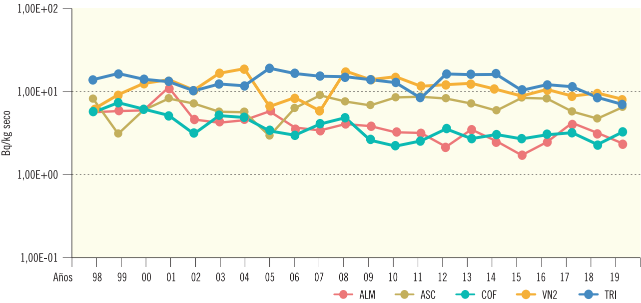
Figura 2.11a. Suelo. Evolución temporal de la concentración de actividad de Cs-137 Valores medios en la zona vigilada
