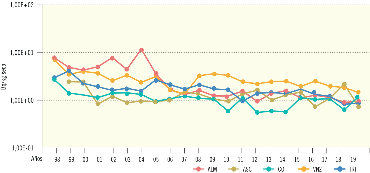
Figura 2.10a. Suelo. Evolución temporal de la concentración de actividad de Sr-90 Valores medios en la zona vigilada
