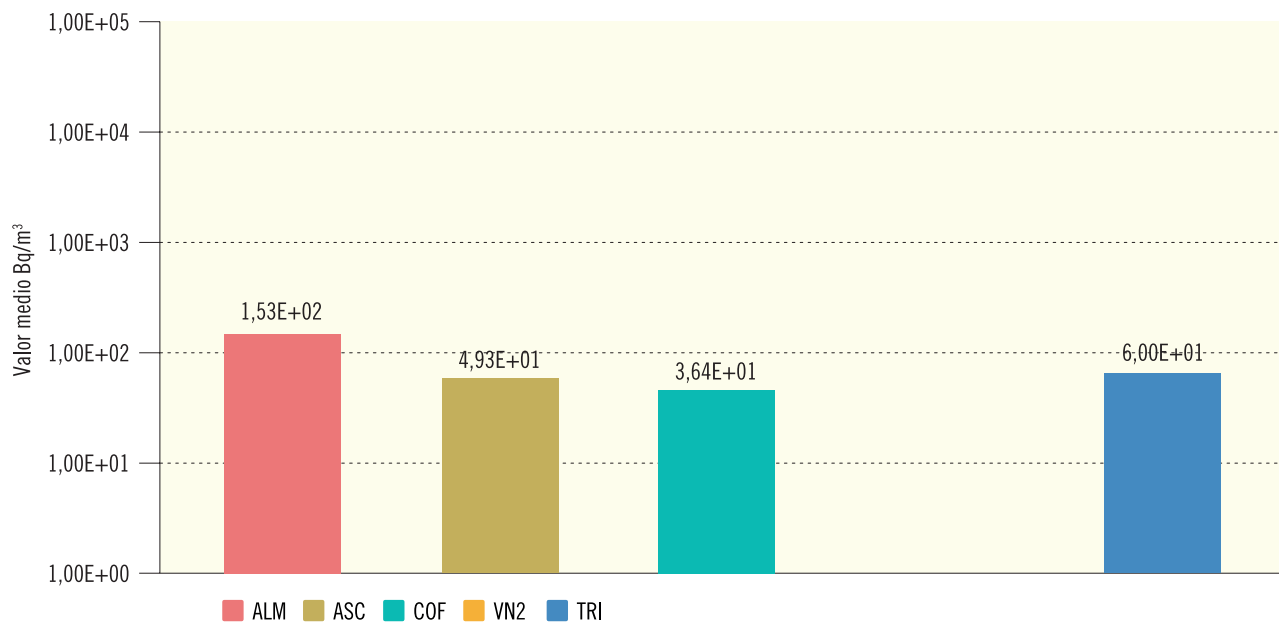
Figura 2.16b. Agua potable. Concentración del índice de actividad beta total (Bq/m³)
