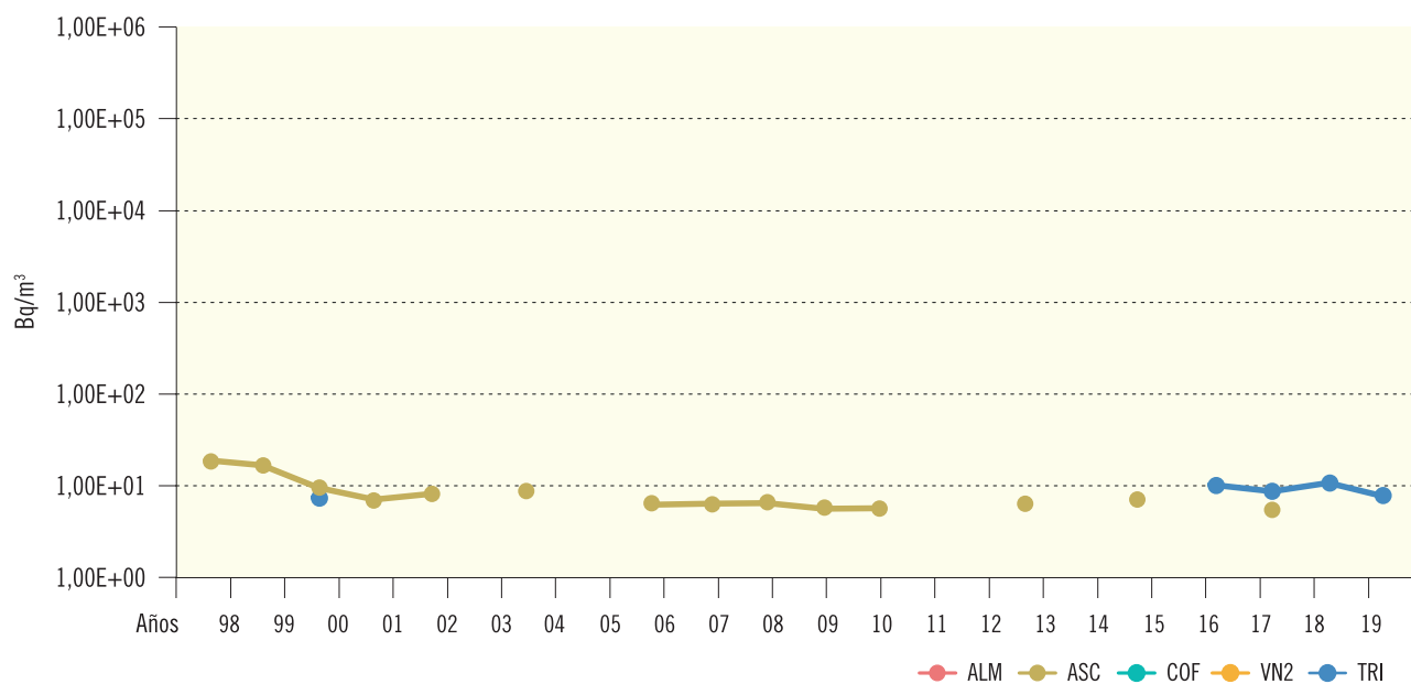
Figura 2.18a. Agua potable. Evolución temporal de la concentración de actividad de Sr-90
