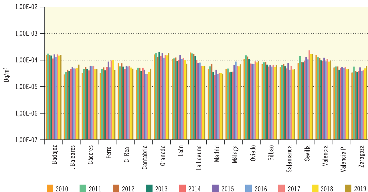
Figura 3.2b. Partículas de polvo en aire. Concentración del índice de actividad alfa total (Bq/m³)
