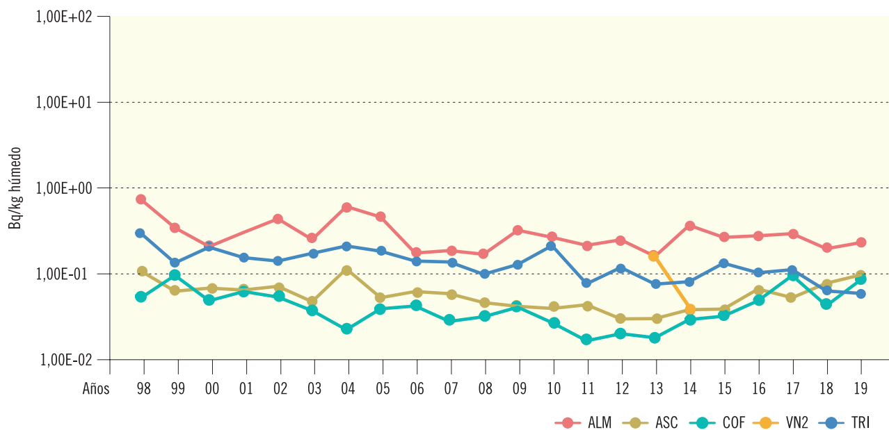
Figura 2.27a. Vegetales de hoja ancha. Evolución temporal de la concentración de actividad de Sr-90
