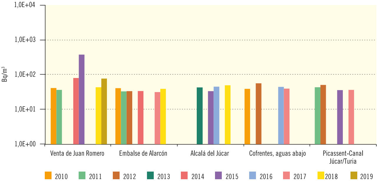
Figura 3.52. Río Júcar Evolución temporal del índice de actividad beta resto
