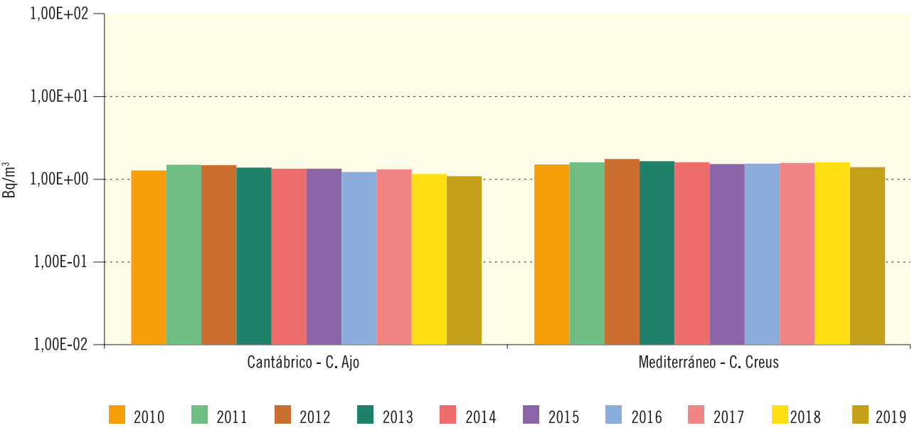
Figura 3.68a. Red de alta sensibilidad. Agua de mar Evolución temporal de la actividad de Cs-137
