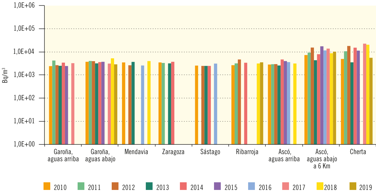
Figura 3.57. Río Ebro Evolución temporal de concentración de actividad de H-3
