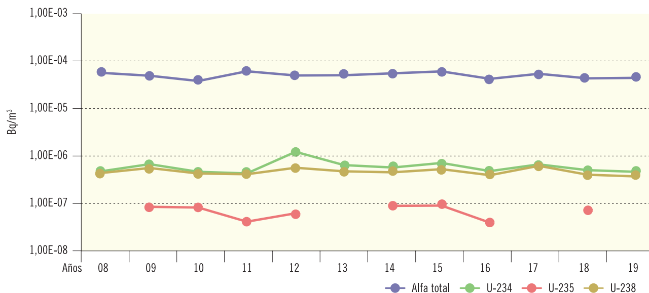
Figura 2.32. Juzbado. Partículas de polvo en aire. Valores de concentración de actividad (Bq/m³)
