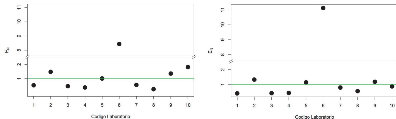
Figura 12. Parámetros E_N calculados para las exposiciones I (gráfico izquierda) y II (gráfico derecha) para cada participante en la intercomparación (Código Laboratorio). En cada gráfico se indica también el intervalo del criterio E_N \leq 1 (línea verde)
