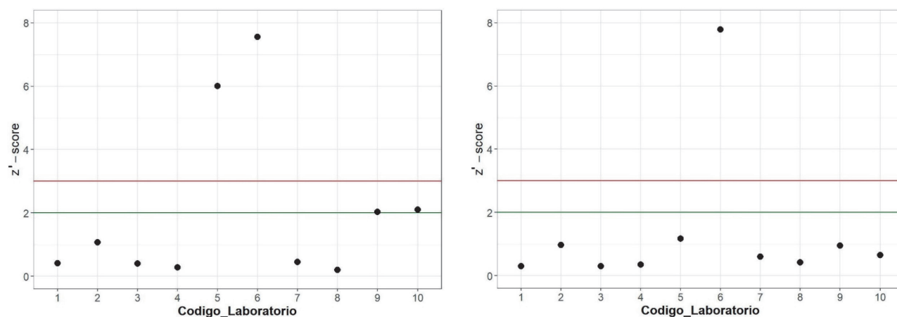
Figura 11. Parámetros z' -score calculados para las dos exposiciones I (gráfico izquierda) y II (gráfico derecha) para cada participante en la intercomparación (Código Laboratorio). En cada gráfico se indican también los intervalos del criterio z' \leq 2 (línea verde) y z' \geq 3 (línea roja)
