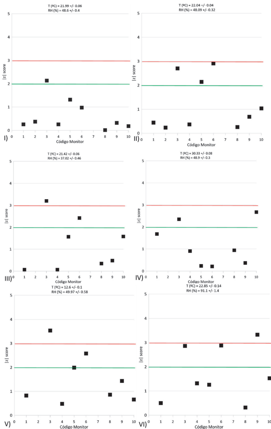
Figura 6. Parámetros z-score (cuadrados negros) calculados para cada una de las exposiciones desde la I a la VI y para cada equipo participante en la intercomparación (Código Monitor). En cada gráfico se indican también los intervalos del criterio |z| \leq 2 (línea verde) y |z| \geq 3 (línea roja)
