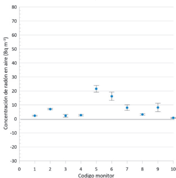
Figura 4. Valor medio de la concentración de fondo medidas por cada monitor continuo durante la exposición VIII
