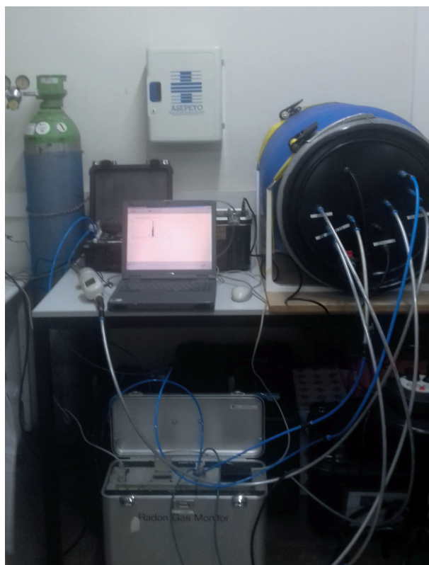
Figura 3. Fotografía del dispositivo montado para llevar a cabo exposición de la fase 3 en la cámara de fondo de radón del INTE-UPC
