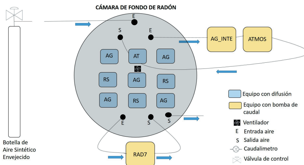
Figura 2. Esquema de la cámara de fondo de equipos de radón del INTE-UPC y configuración utilizada durante la fase 3
