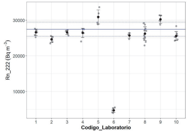
Figura 10. Valores medios y desviaciones estándar de la concentración de radón medida en la cámara STAR del INTE-UPC durante las exposiciones I y II de la tabla 7. El valor medio medido por el equipo de referencia (línea azul) y su incertidumbre expandida (líneas discontinuas) se presentan también
