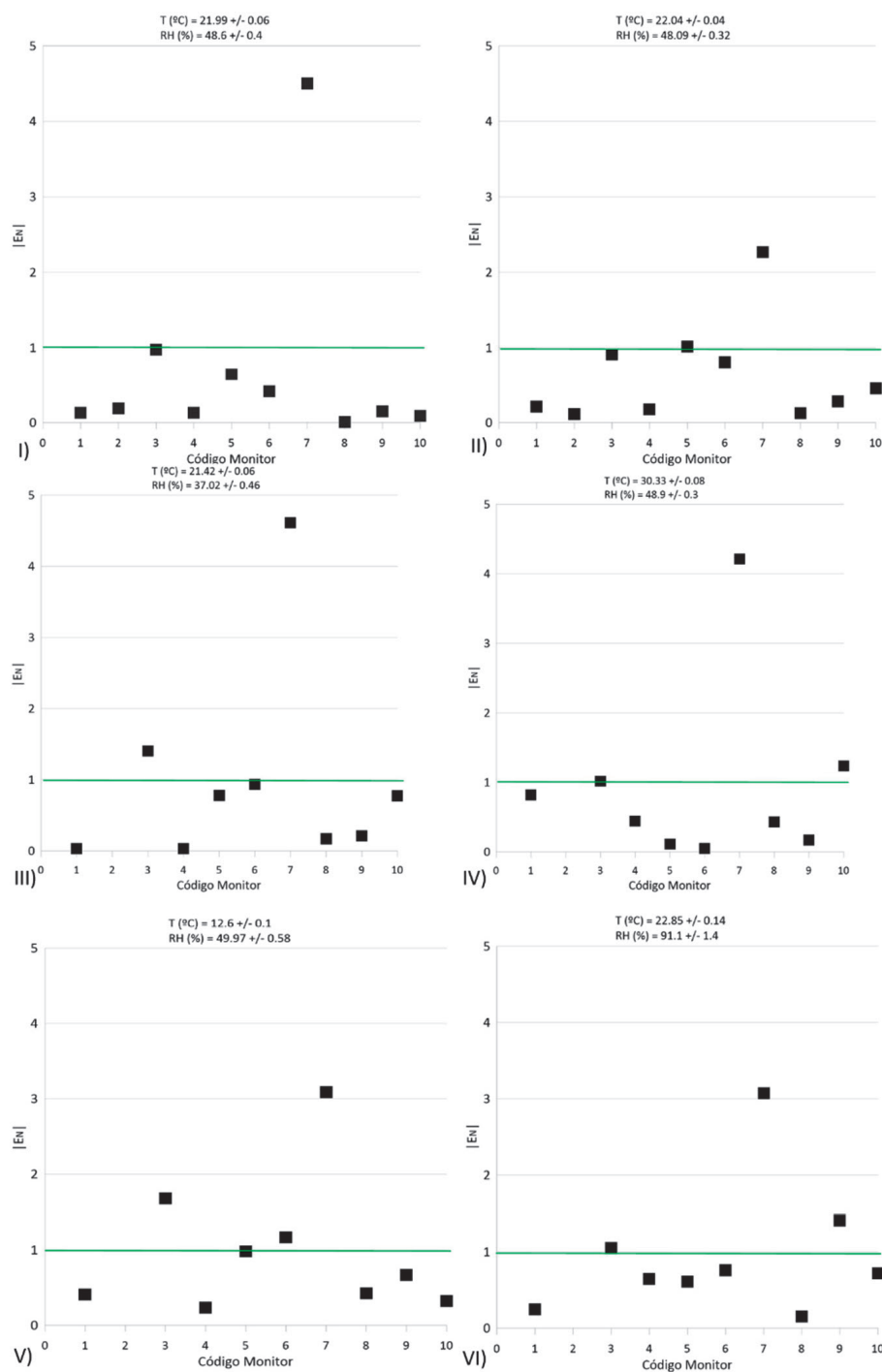
Figura 7. Parámetros E_N (cuadrados negros) calculados para cada una de las exposiciones desde la I a la VI y para cada equipo participante en la intercomparación (Código Monitor). En cada gráfico se indica también el intervalo del criterio |E_N| \leq 1 (línea verde) y las condiciones ambientales bajo las cuales se ha llevado a cabo la medida
