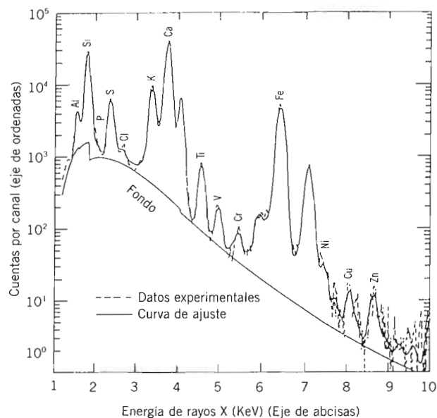
Figura 6: Espectro típico de rayos X tras emplear la técnica de P.I.X.E. en una muestra de petróleo de esquisto.
