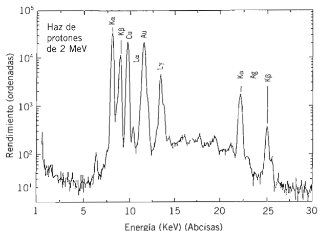
Figura 7: Espectro de P.I.X.E.
