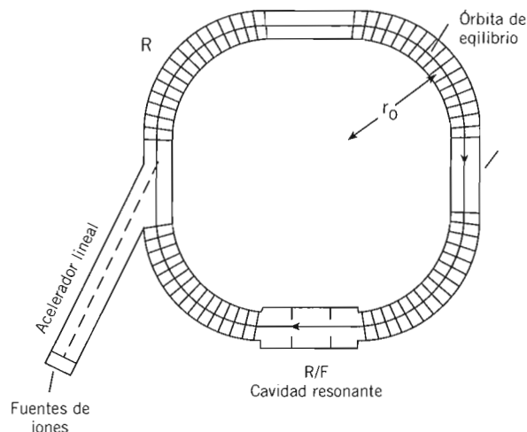
Figura 5: Cámara de vacío compuesta por cuatro secciones magnéticas en régimen pulsado.
