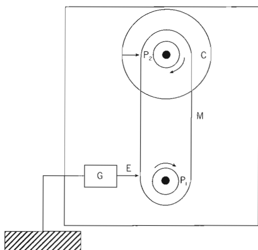
Figura 2-1: Esquema del generador Van de Graaff.
