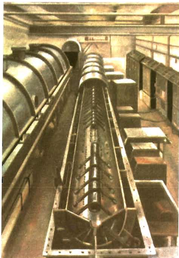
Figura 4: Acelerador lineal de protones del CFIRN. 50 MeV.
