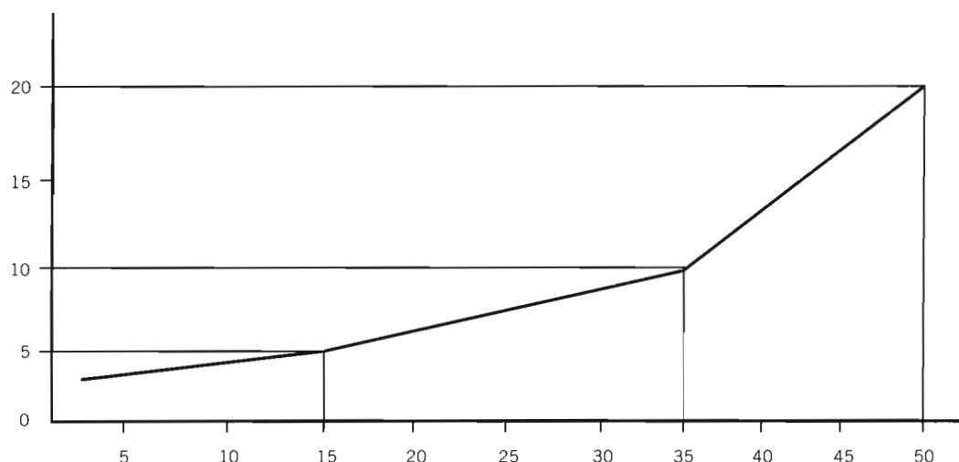
Figura 25. Limitación de la radiación parásita en un haz de electrones. En ordenadas está representado el % de dosis absorbida que no debe sobrepasarse 100 mm más allá del alcance práctico de los electrones.
