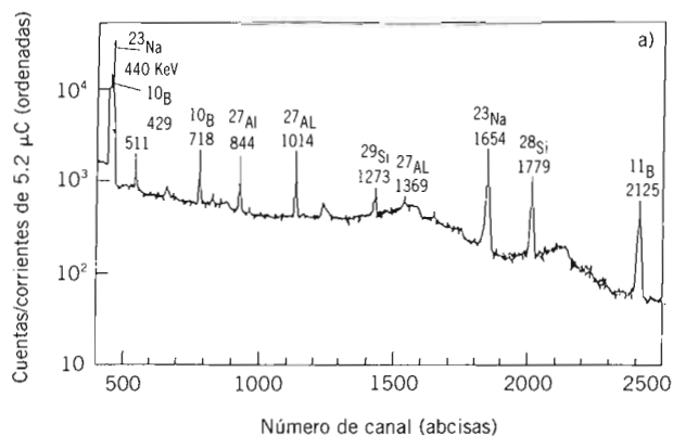
Figura 8: Espectro de P.I.G.E. de una muestra de vidrio contemporáneo.
