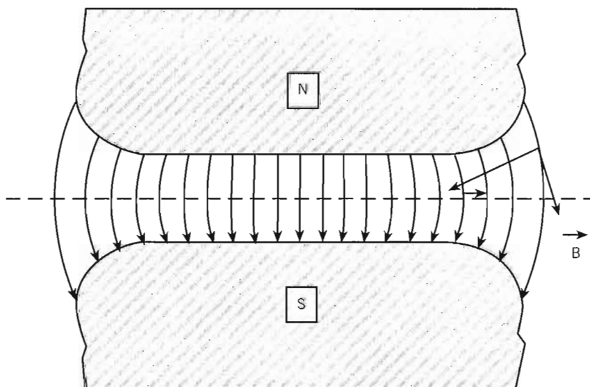
Figura 2: Perfil de piezas polares en un ciclotrón clásico
