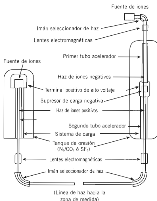
Figura 3. Componentes de un sistema de aceleración de iones: 1. Fuente de iones; 2. 1 a etapa simple; 3. 2 a etapa simple (tándem); 4. 3 a etapa simple (tándem)
