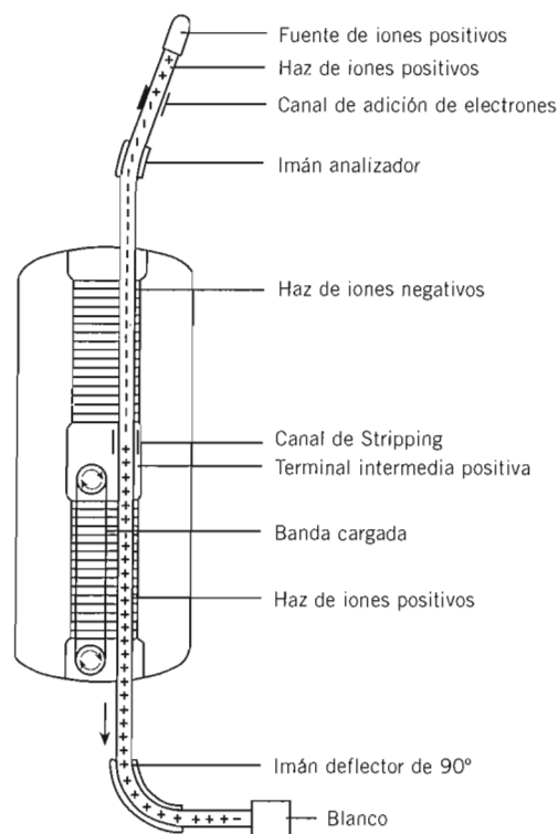
Figura 2: Principio de operación de un acelerador tándem Van de Graaff
