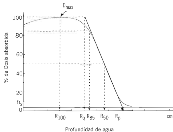
Figura 1: Curva de distribución de dosis absorbida en profundidad. Electrones de 16 MeV de energía nominal. Campo de 20 x 20 cm a 100 cm de DFS. Se muestran la profundidad del máximo de dosis y los alcances R_{85} y R_p definidos en el texto.
