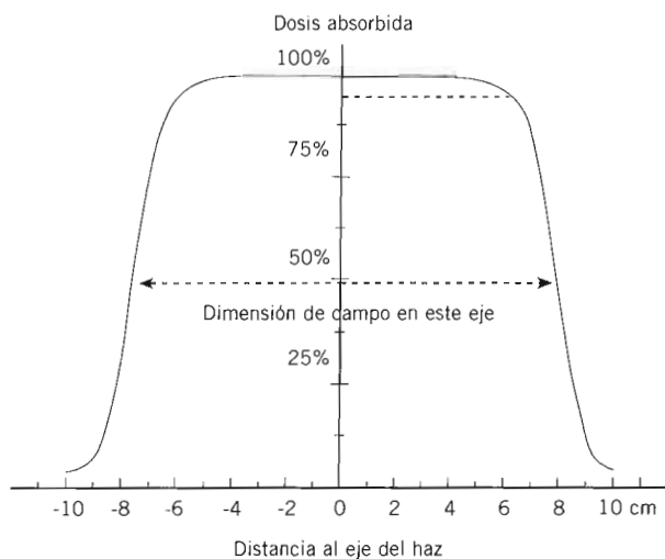
Figura 4: Distribución de dosis absorbida a lo largo de un eje del campo de radiación a la profundidad del máximo de dosis. Electrones de 12 MeV. Campo de 15 \times 15 cm 2 a D.F.S. 100 cm.
