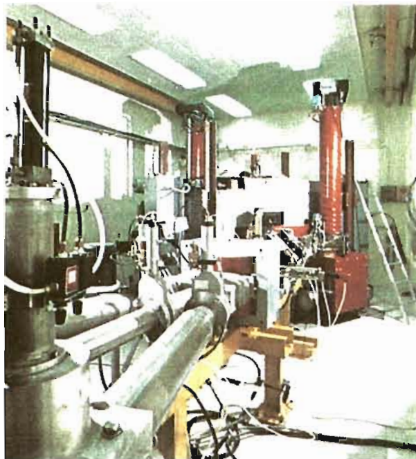
Figura 5: Ciclotrón del Servicio Hospitalario Frédéric Joliot (CEA-Francia).
