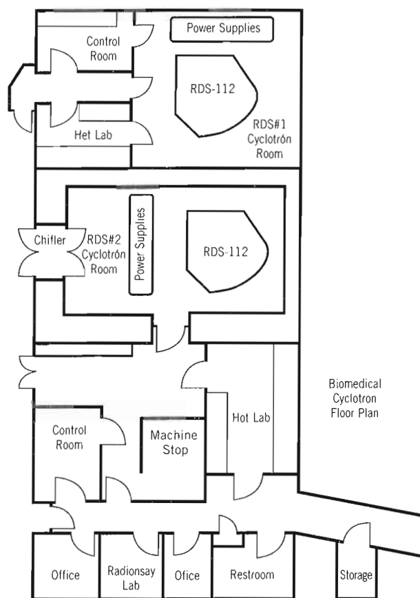
Figura 3. Diagrama de planta del ciclotrón
