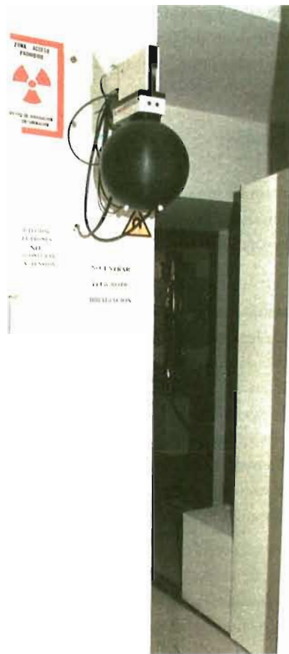
Figura 5: Detector de neutrones a la entrada del bunker del ciclotrón.
