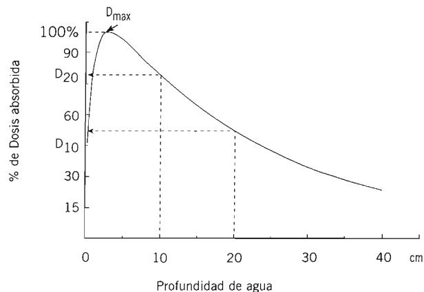
Figura 4. Curva de distribución de dosis a lo largo de la profundidad 10% de 10 MeV. Campo de 10x10 cm 2 a 100 cm de DFS.
