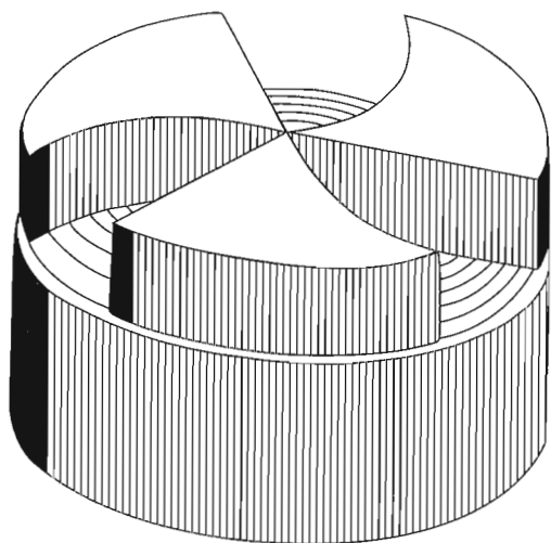
Figura 6: Perfil de pieza polar en un ciclotrón isocrono.
