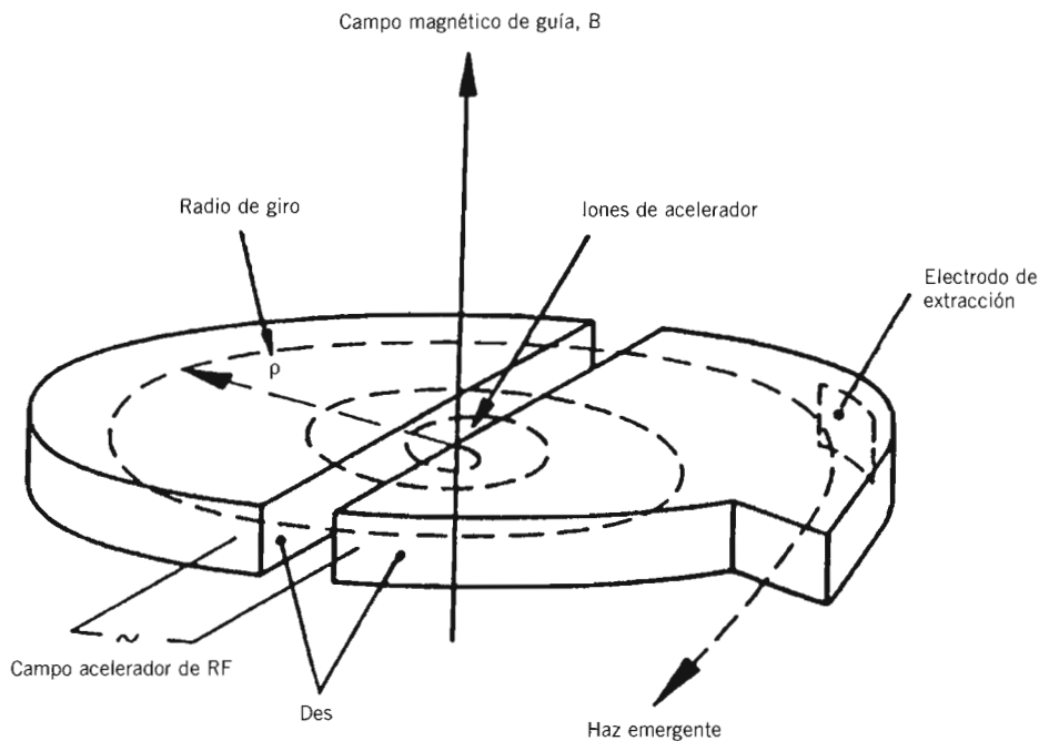
Figura 1: Esquema de un Ciclotrón
