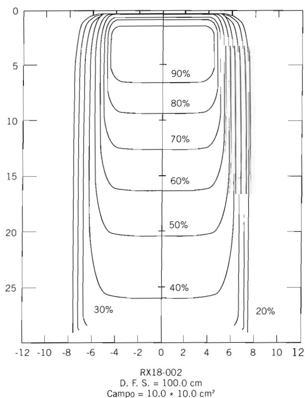
Figura 5: Distribución de dosis en un plano que contiene el eje del haz. RX 18 MV. Campo de 10 \times 10 cm 2 a D.F.S. 100 cm.
