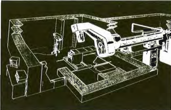
Figura 3: Esquema de blindajes en sala de tratamiento con acelerador lineal.
