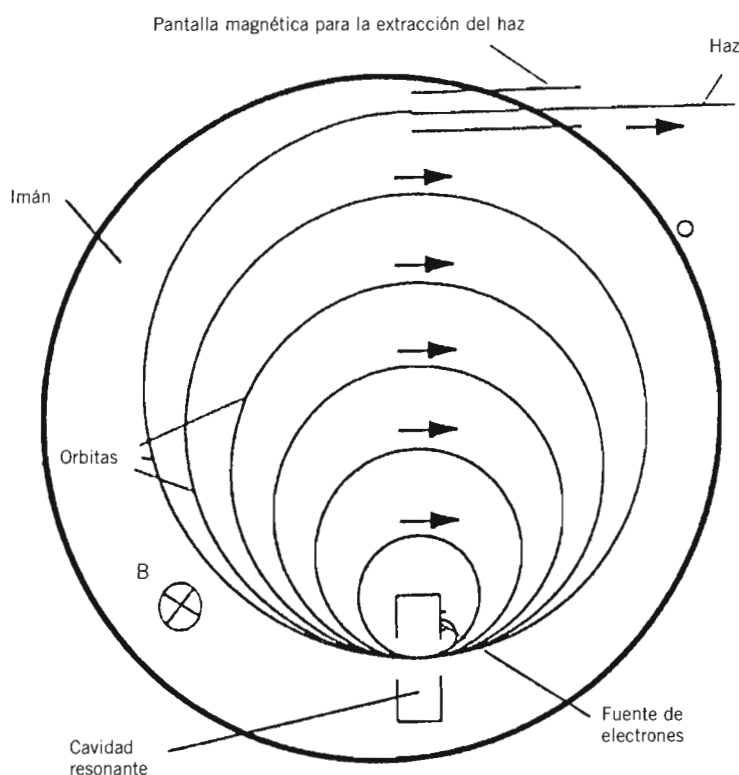
Figura 3: Esquema fundamental de un microtrón.
