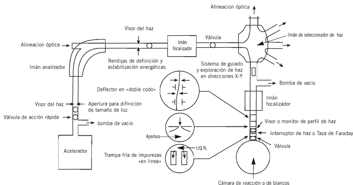
Figura 4: Sistema de transporte del haz.
