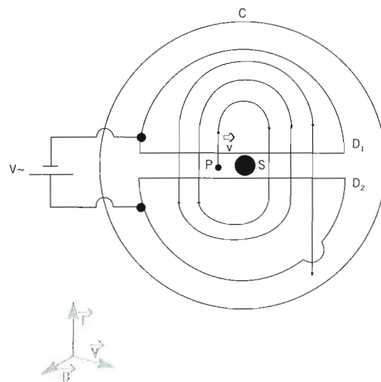
Figura 3: Esquema del Ciclotrón
