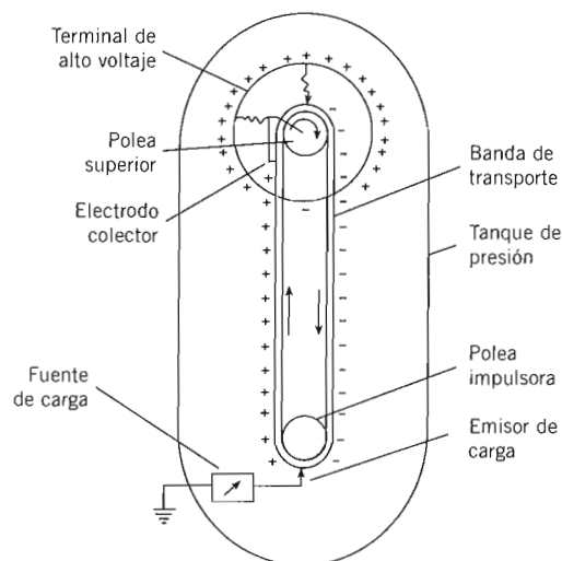
Figura 1: Esquema del mecanismo interno de un acelerador Van de Graaff.
