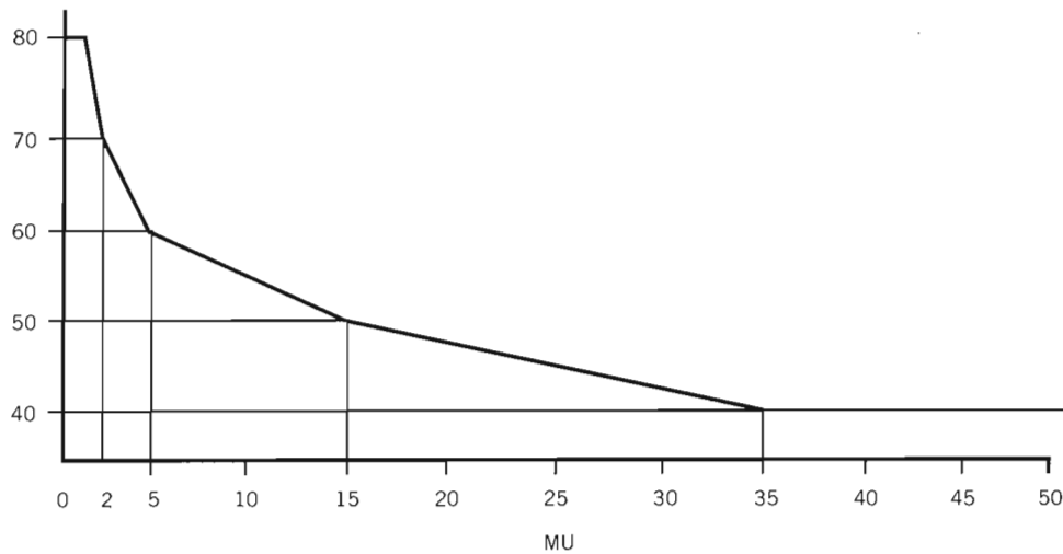
Figura 26. Limitación de la dosis absorbida en superficie durante la irradiación con R. X.
