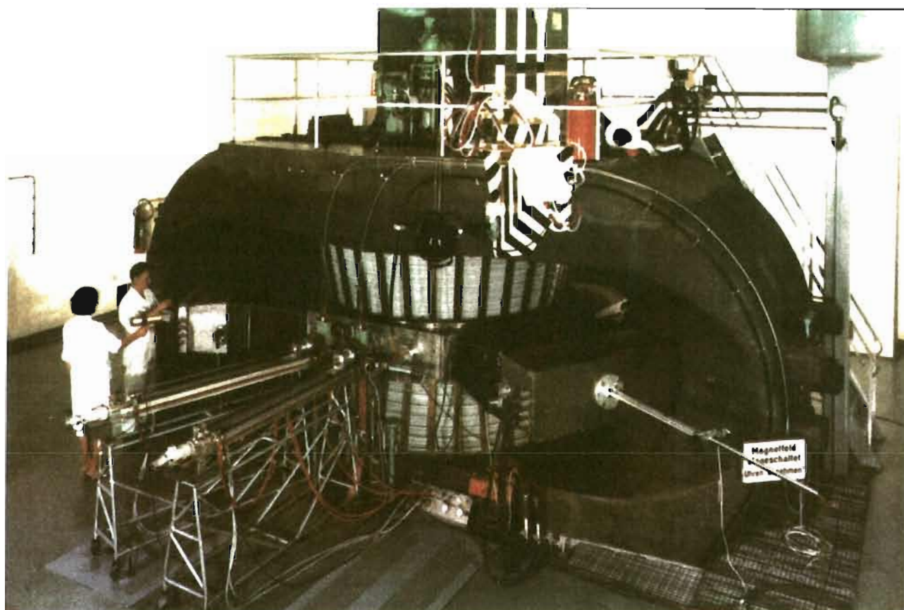
Figura 3. Aceleración de RER 100 MeV (Fuente: OIEA, 1995, p. 100)
