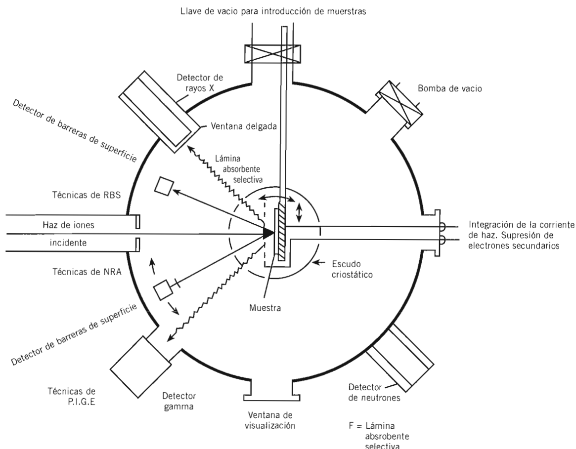
Figura 5: Cámara de blancos esquemática para análisis de haces de iones de alta energía.
