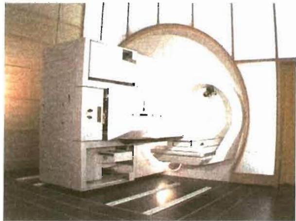
Fig. 4.10. Ciclotrón superconductor.
