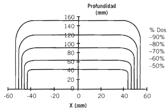
Figura 7a. Plano que contiene al eje del haz
