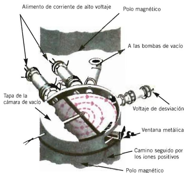
Figura 2: Esquema de un ciclotrón
