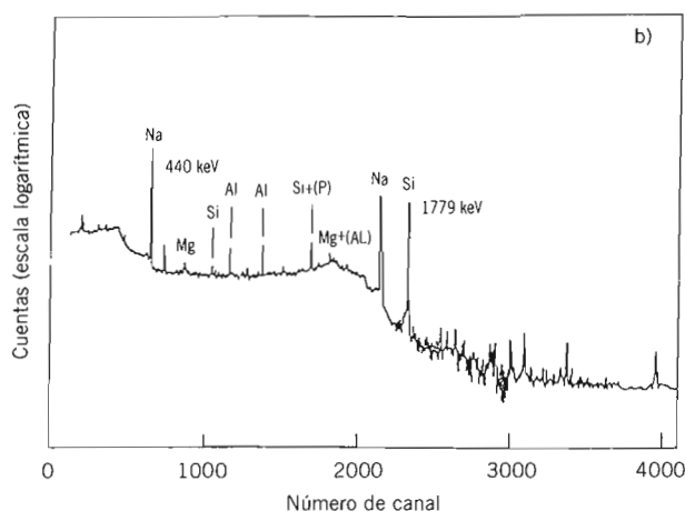
Figura 9: Espectro de P.G.E. de una muestra de vidrio del imperio romano tardío.
