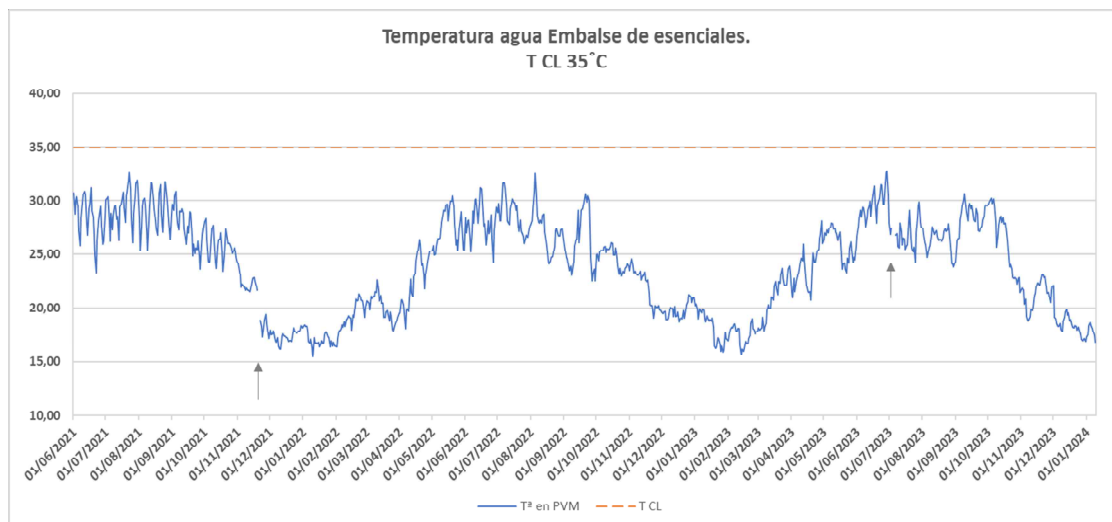
Figura 2: temperaturas medidas en el agua del Embalse de servicios esenciales.
