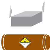
Aplastamiento: caída de plancha de 500 kg desde 9 m (para bultos de peso y densidad bajos)
