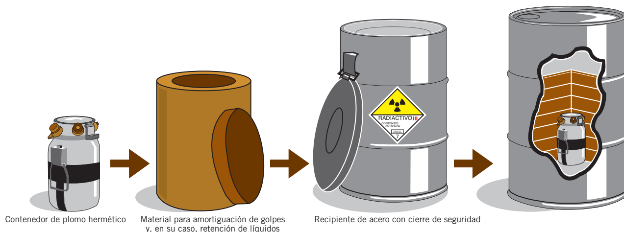
Ejemplo de bulto tipo B.
