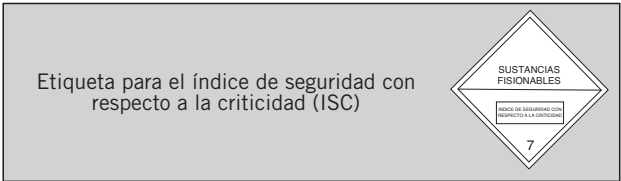
Etiquetado de bultos radiactivos para su transporte.
