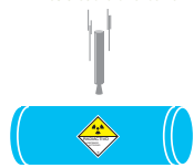
Desgarramiento: caída de barra de 250 kg desde 3 m (peso del bulto < 250 kg)
