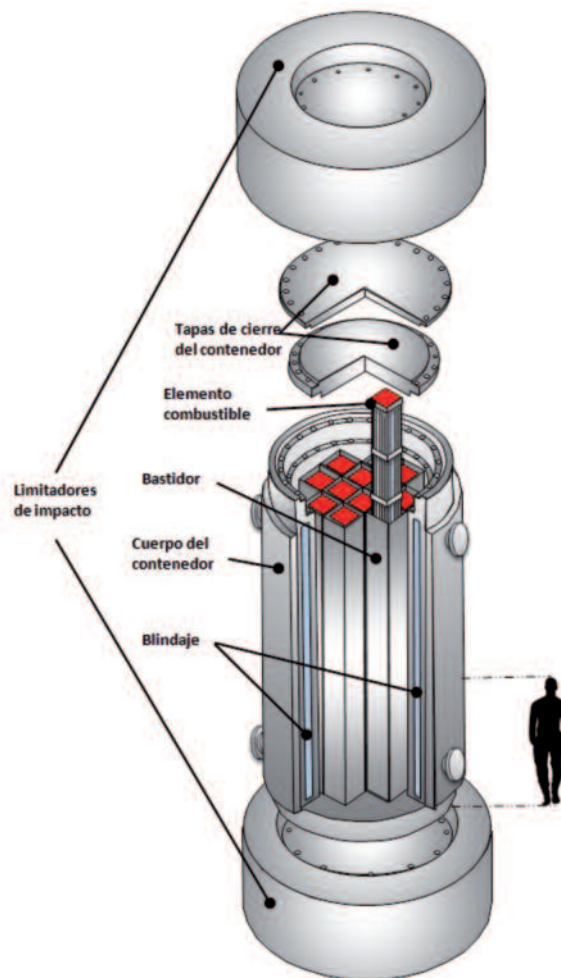
Ejemplo de bulto para combustible irradiado
