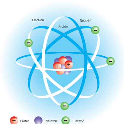
Estructura del átomo.
