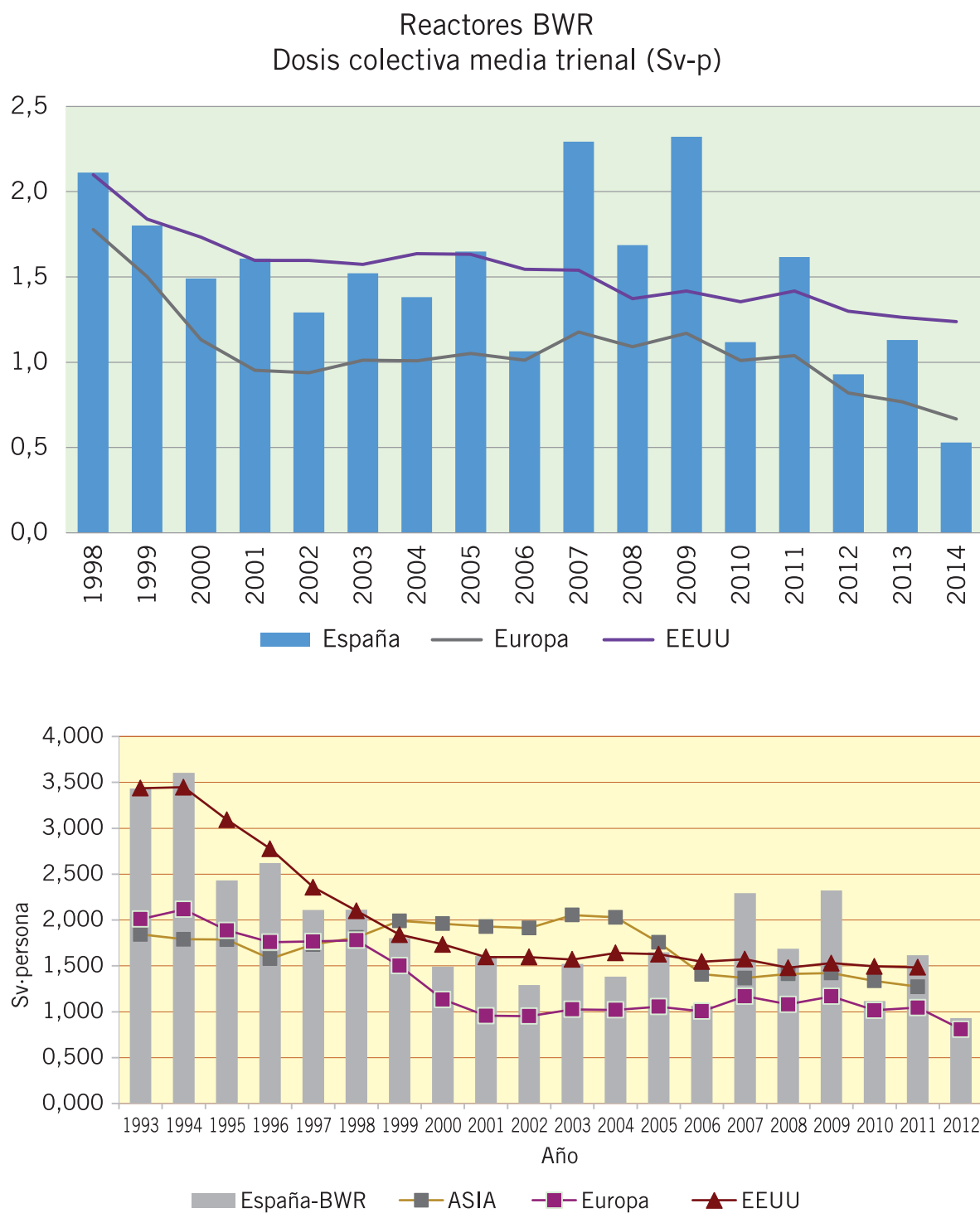
Figura 15.A.2. Dosis colectiva trienal media (Sv.persona) para reactores de tipo BWR. Comparación internacional.
