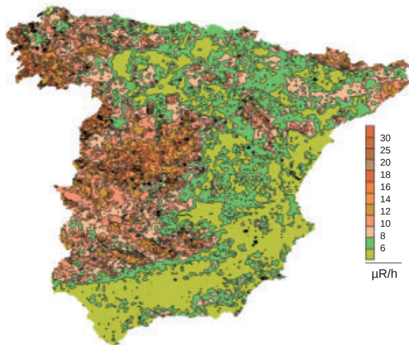
Niveles de tasa de exposición a la radiación gamma natural medidas a un metro del suelo correspondiente a la España peninsular.
