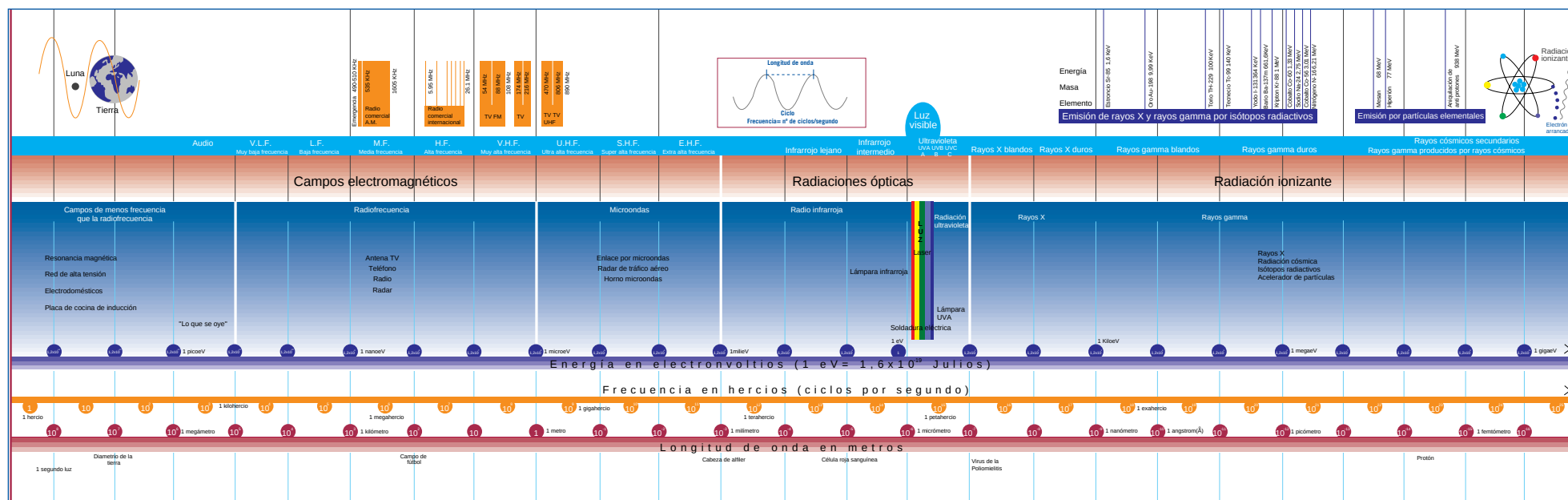
Espectro de ondas electromagnéticas
