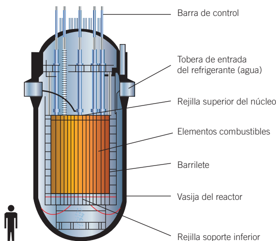
Esquema de un reactor nuclear PWR
