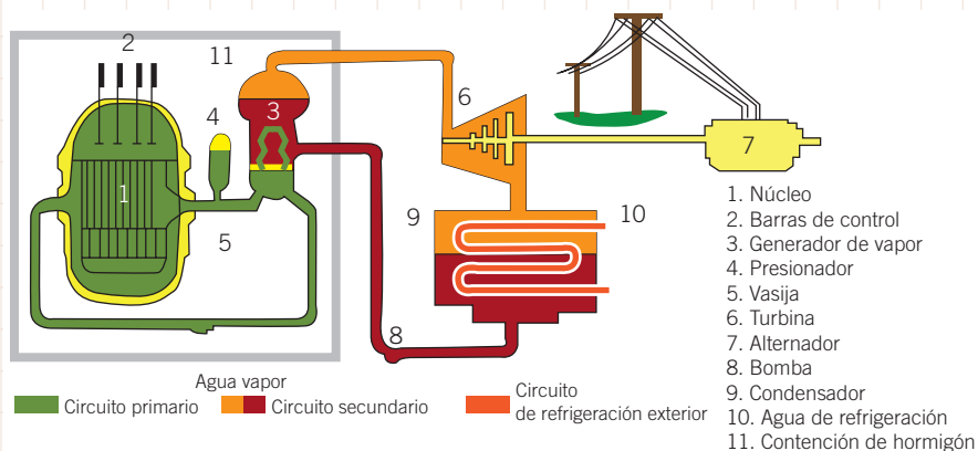
Esquema de una central de agua a presión
