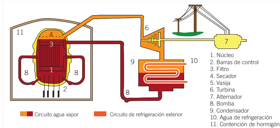
Esquema de funcionamiento de una central nuclear (BWR)
