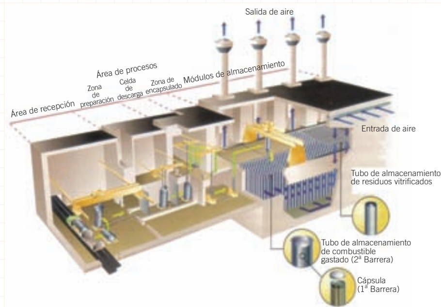
Esquema de AIC. Cámaras
