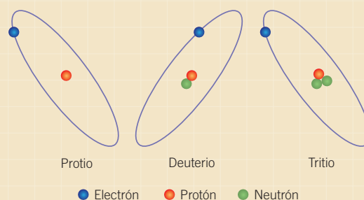
Los tres isótopos del hidrógeno
