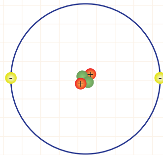
Átomo de helio
