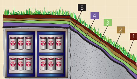
Esquema instalación de almacenamiento en la superficie.
