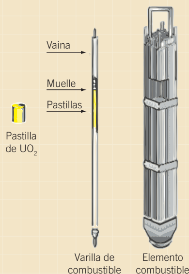
Composición de un elemento combustible
