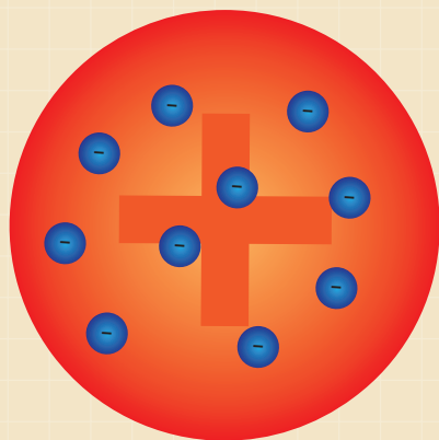
Modelo atómico de Thomson
