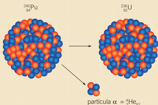
Desintegración del plutonio-240
