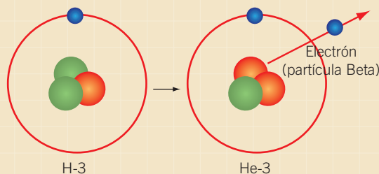
Emisión de una partícula beta
