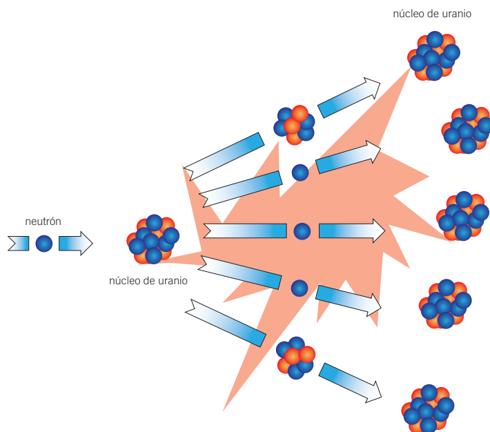
Reacción en cadena
