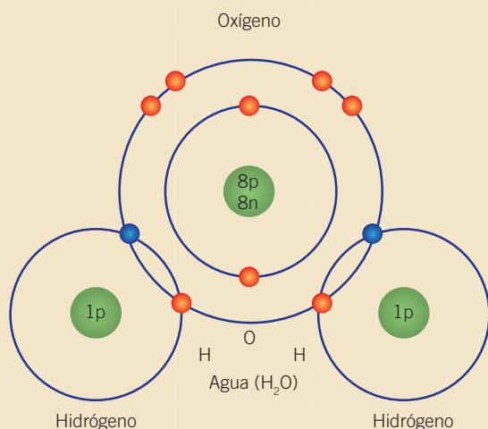
Molécula de agua
