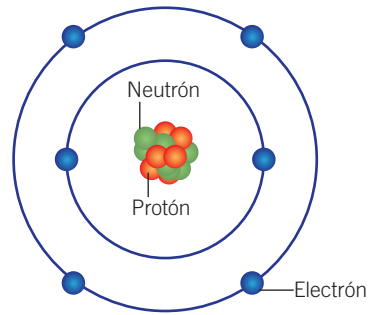
Átomo de carbono
