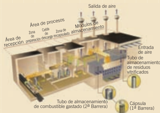
Esquema ATC Camaras
