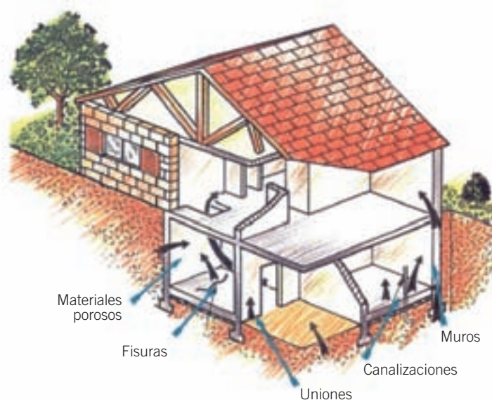
Principales vías de entrada de radón en una casa
