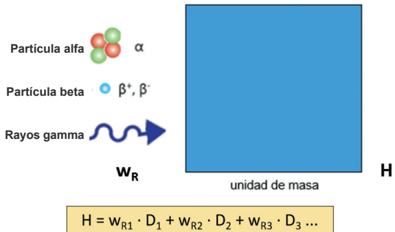
Figura 11. Representación de la dosis equivalente en el caso de incidencia simultánea de distintos tipos de radiación.
