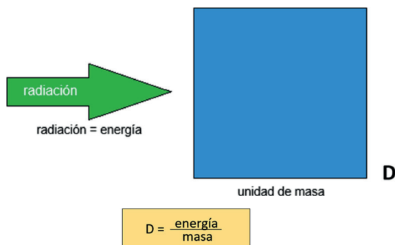
Figura 10. Representación de la dosis absorbida.
