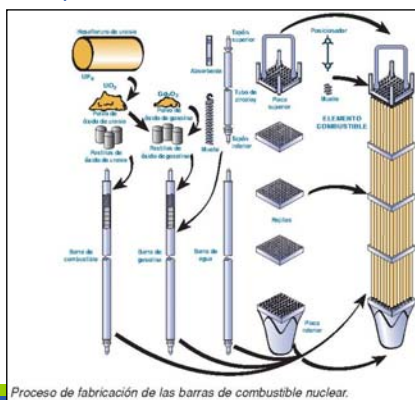
Proceso de fabricación de las barras de combustible nuclear.
