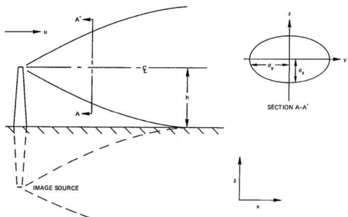
Figura 6 Diagrama dispersión de penacho Gaussiano
