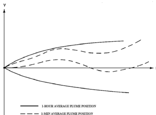
Figura 1. Representación del penacho instantáneo y su envolvente como promedio en una hora
