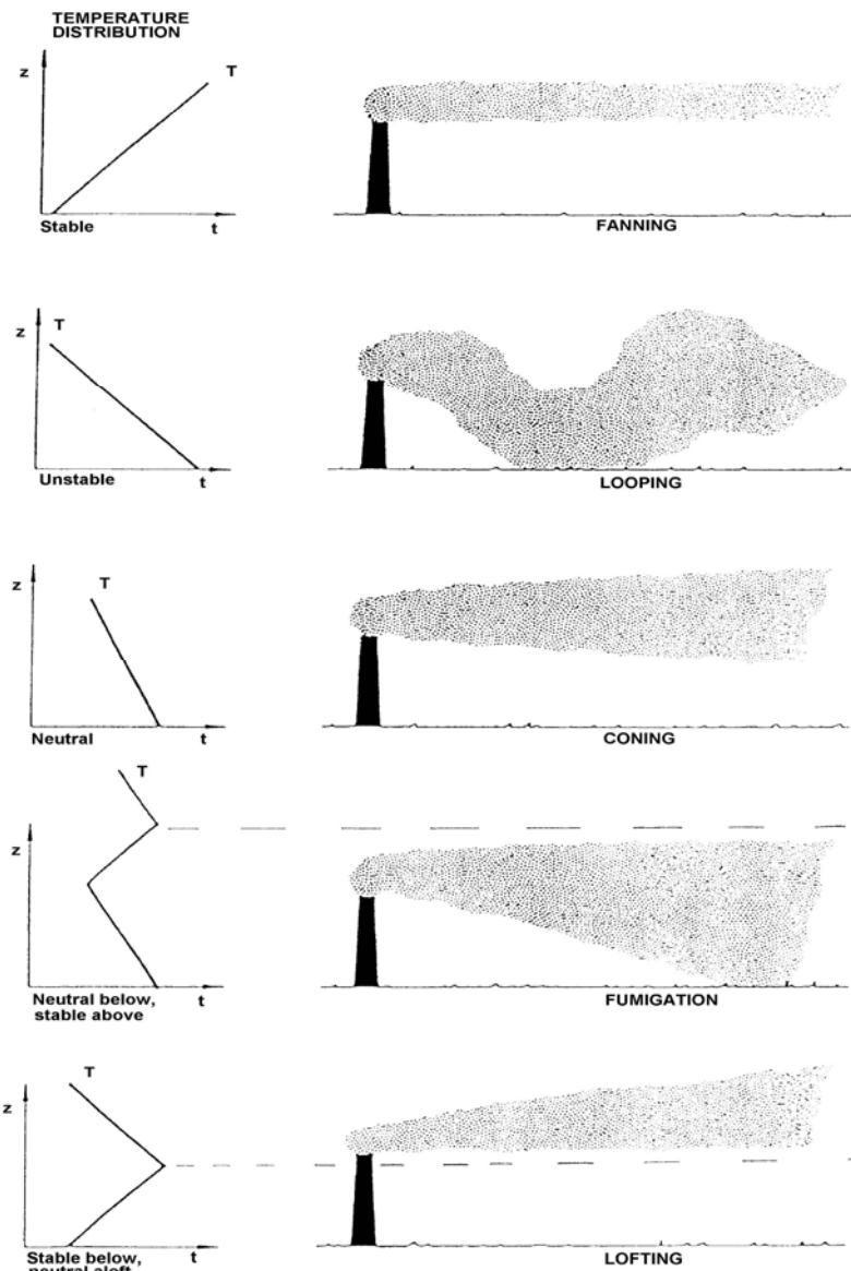
Figura 5. Varios tipos de pautas de penacho dependiendo de los perfiles de temperatura.
