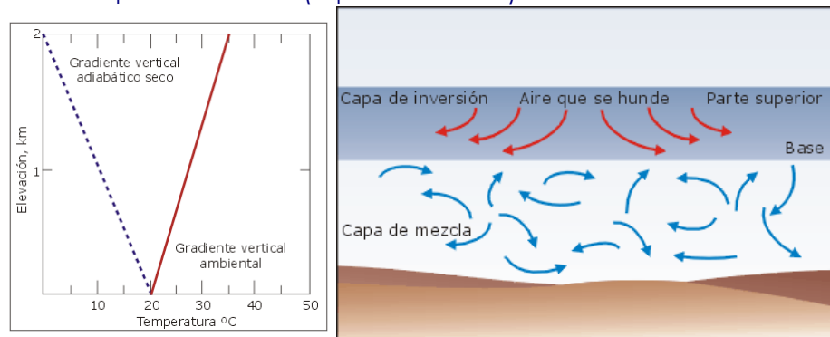
Figura 3. Inversión Térmica.
