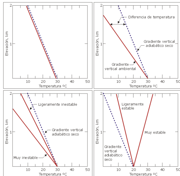
Figura 2. Gradiente adiabático seco. Condiciones atmosféricas.
