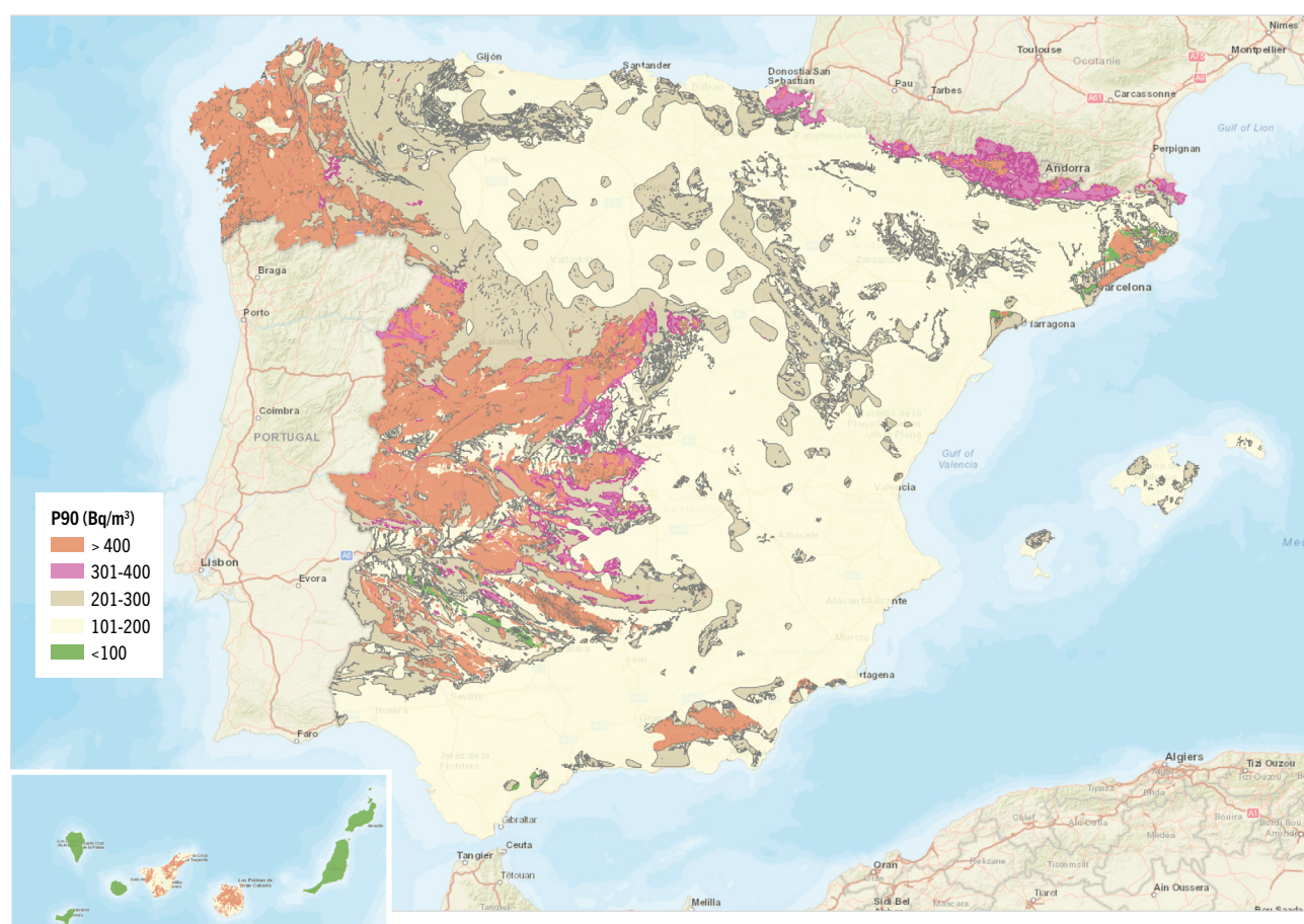
Figura 5.2.2.1. Mapa del potencial de radón de España
