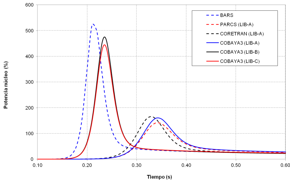
Análisis de una expulsión de barra de control
